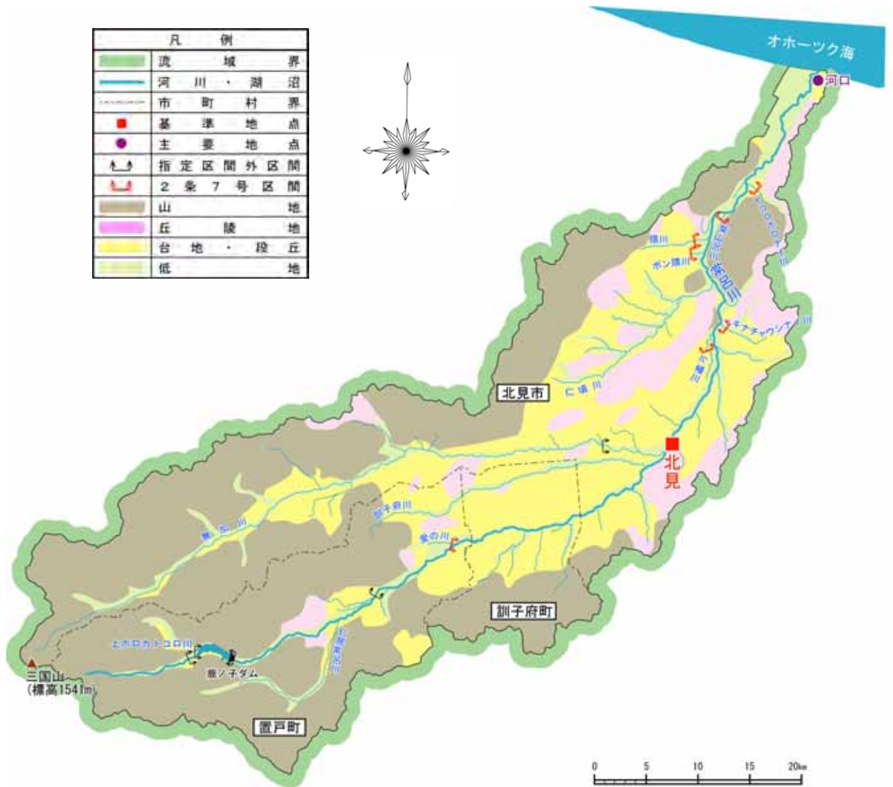
図 1-2 地形図
