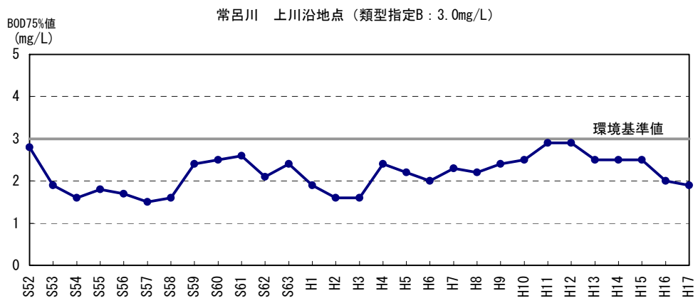
図 1-14 水質(BOD75%値)の経年変化
