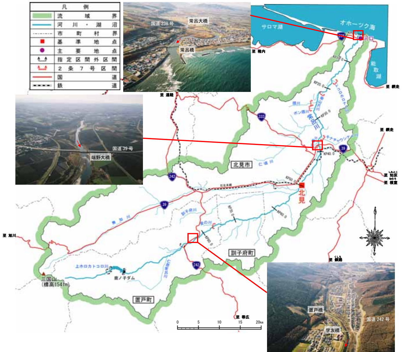
図 1-4 基幹交通施設位置図
