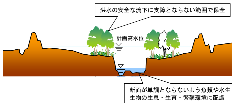
図 2-6 河畔林の保全、河岸の多様化イメージ図
