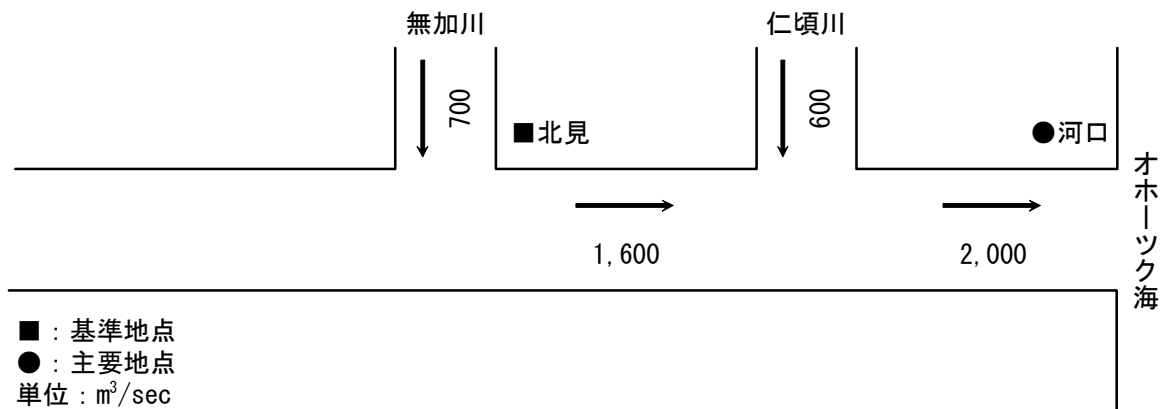
図 1-8 常呂川水系河川整備基本方針における常呂川計画高水流量配分図
