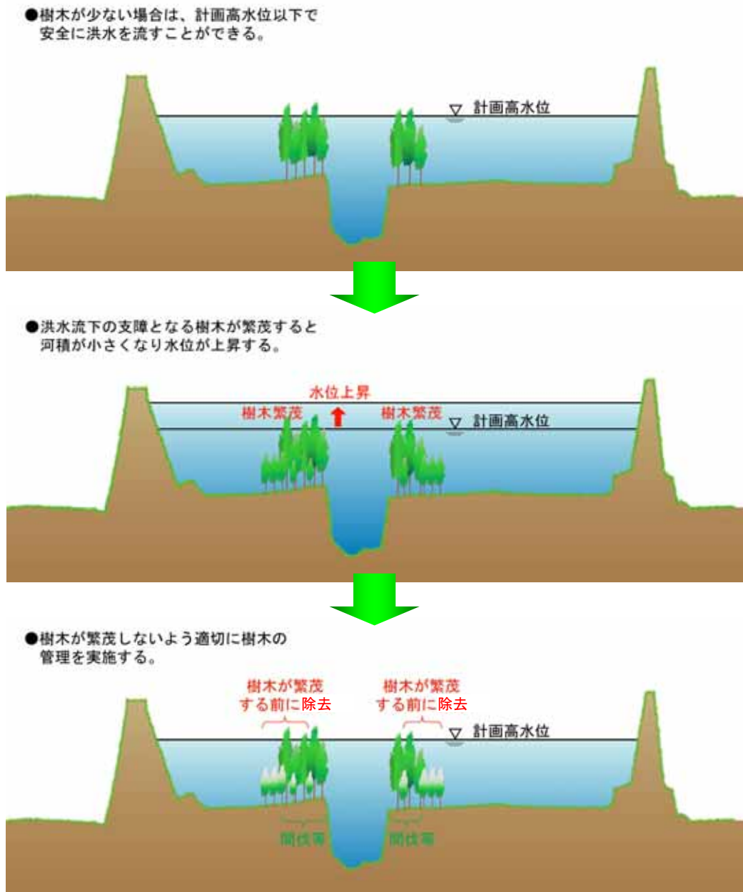
図 2-10 河道内樹木の保全イメージ図
