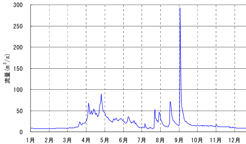
図 1-11 日平均流量の年変化(常呂川 北見地点 平成 17 年)
