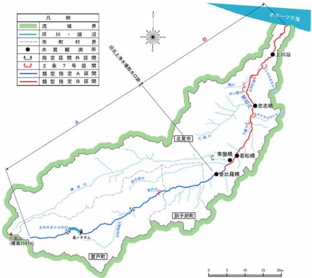
図 1-13 水質環境基準の類型指定区間
