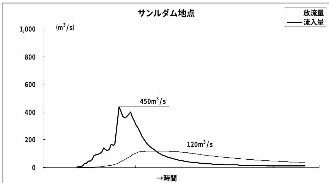
図-2 ハイドログラフ
