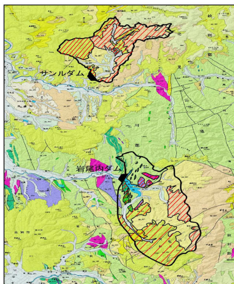
火成岩類
