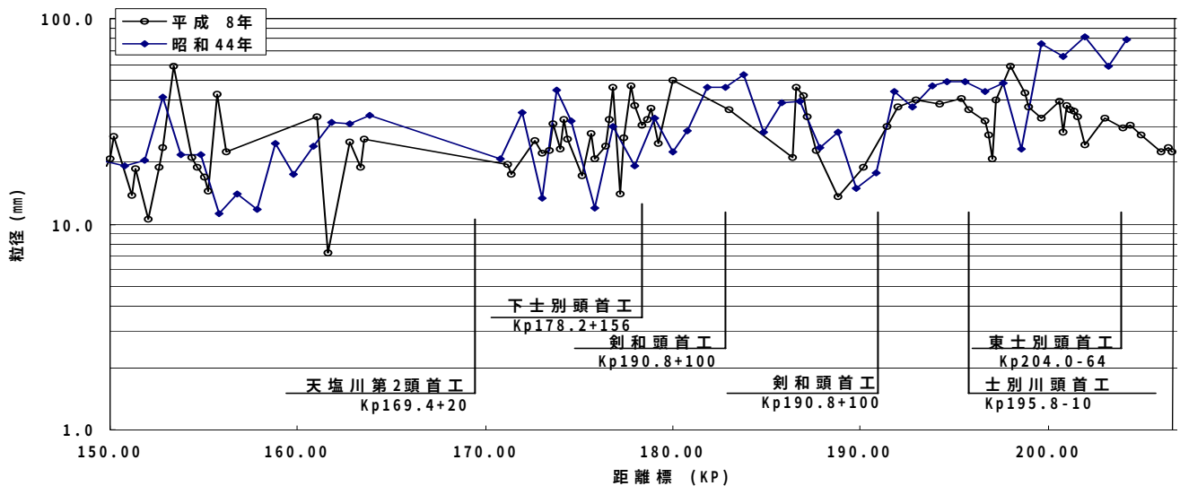
図-6 河床材料の経時変化
