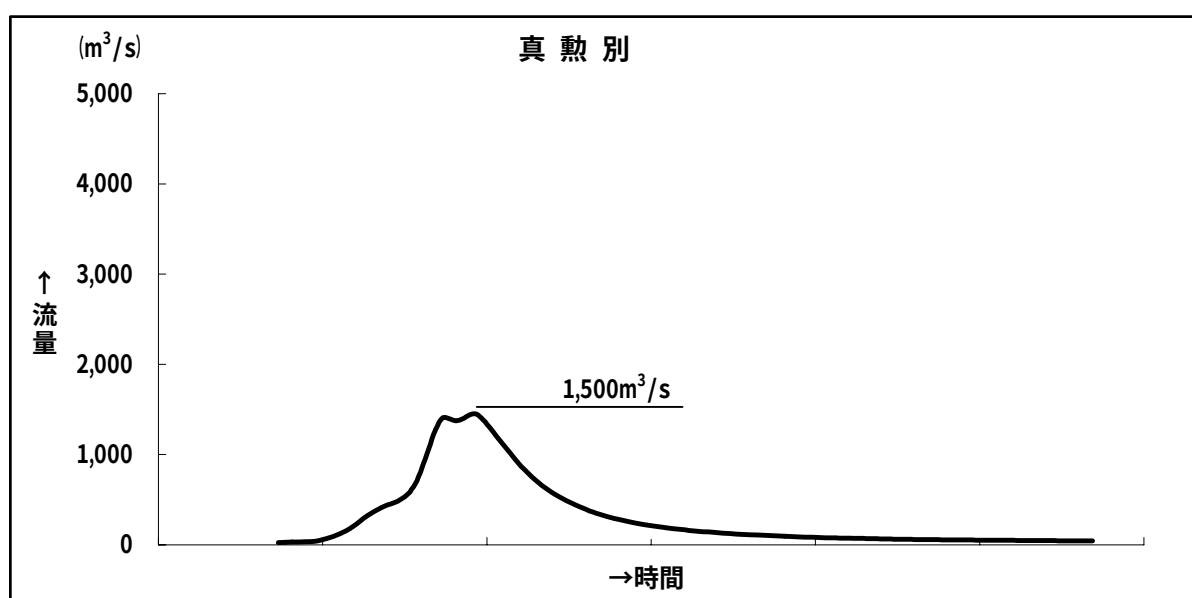
図ー1 整備計画目標ハイドログラフ*(昭和48年8月型)
