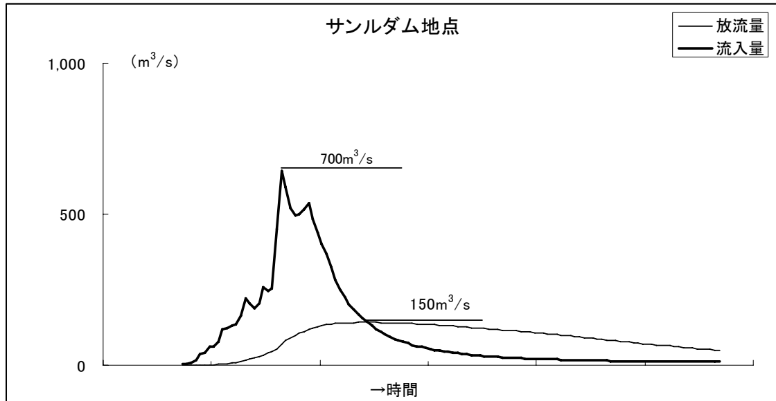
図-1 基本方針目標流量に対するサンルダムの効果
