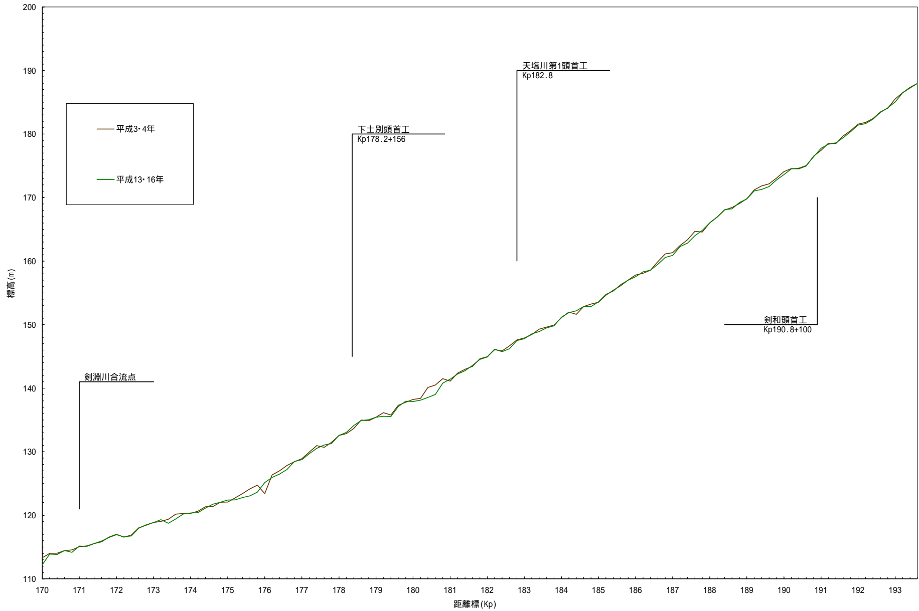
図 - 7 最深河床高の経時変化
