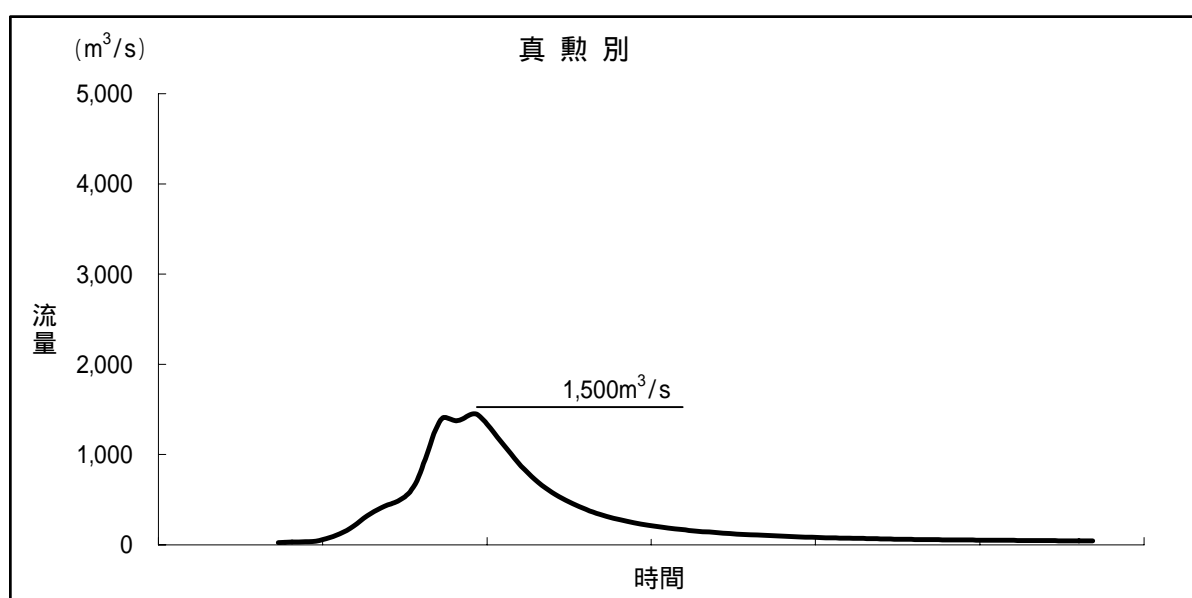
図 - 1 整備計画目標ハイドログラフ* (昭和 48 年 8 月型)
