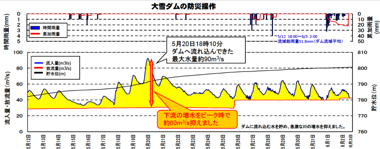
大雪ダム貯水状況
