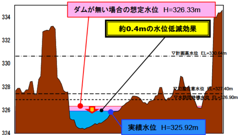
上川水位観測所地点における水位低減効果
