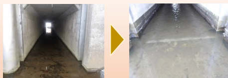
水門堆積土砂撤去(後志利別川・稲穂樋門)
