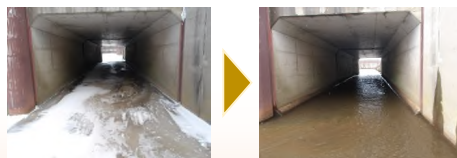
水門堆積土砂撤去(後志利別川・愛知1号樋門)
