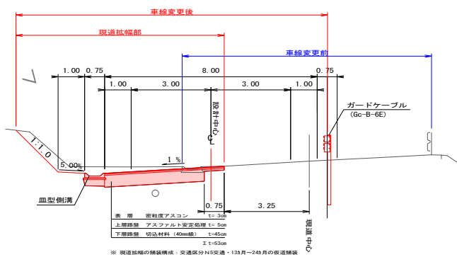
車線変更箇所 断面図
