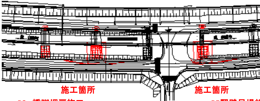
P3 橋脚埋戻し施工
