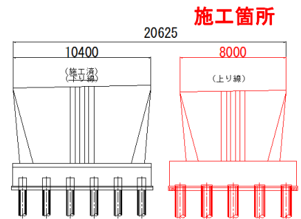
P5 底板コンクリート散水養生
