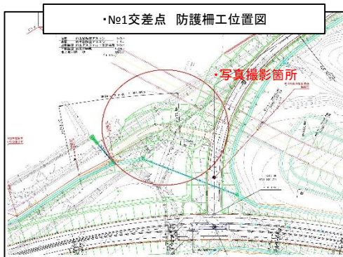
No1交差点 防護柵工
