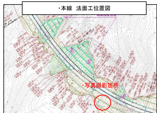
本線 法面工 切土法面整形
