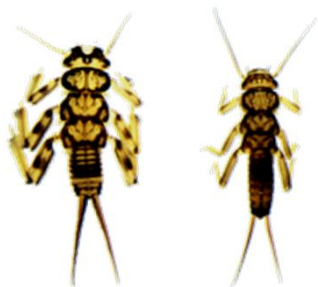
カワゲラ類
