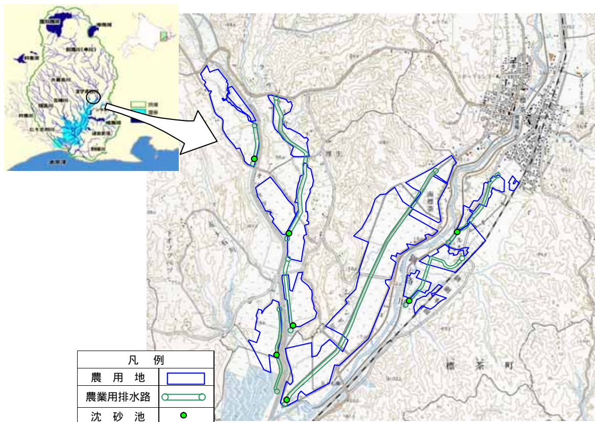
沈砂池設置位置図
