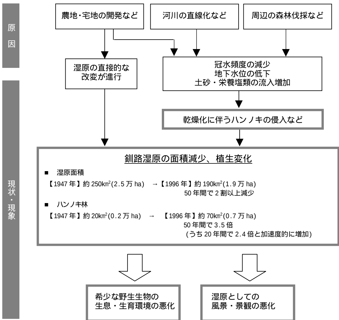
図 2-4 湿原環境変化の要因と現状
