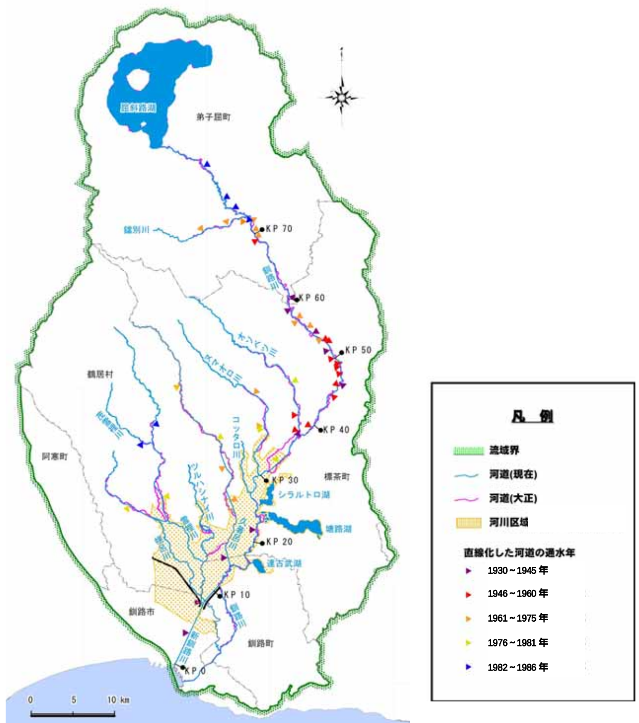
図 2-1 釧路川流域河道変遷図(大正と現在の比較)
