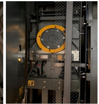
つり合いおもり・巻上機
