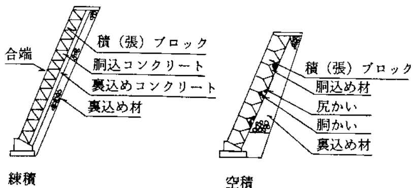
図5-5 コンクリートブロック工
