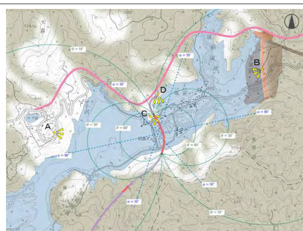
ダム湖を跨ぐ橋梁における視点場分析図。視線入射角、水平見込角、可視不可視領域を示すとともに、地域特性や環境特性を踏まえて、重要になると考えられる視点場を抽出し、考察を加えている。
