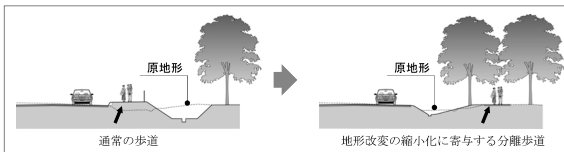
図 7.2 分離歩道構造による地形改変の縮小化
