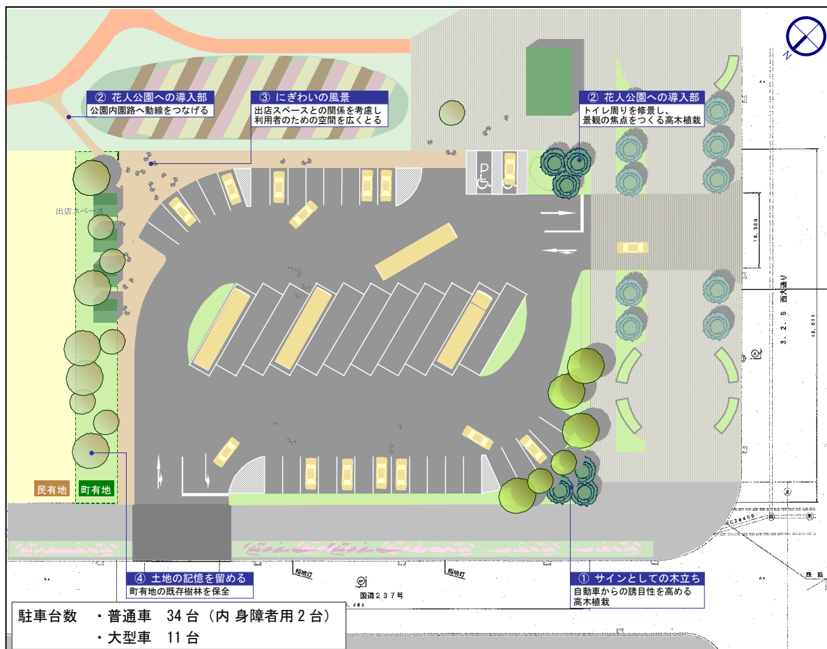
図 5.8.3 計画平面図
