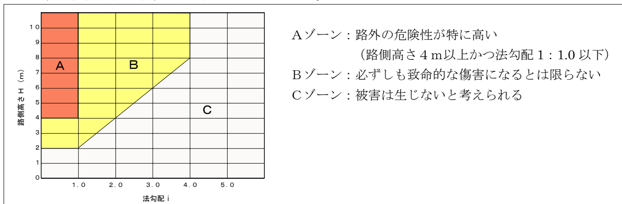
図 9.1 防護柵が必要な法勾配と盛土高さ（出典：資料1）
