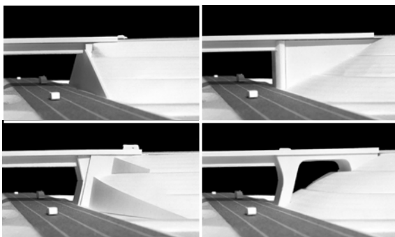
図 5.3.2 モデルによる構造形式検討。左上は予備設計成果、右上は箱式橋台＋盛りこぼし案、左下は二段擁壁で橋台のコンパクト化を図った案、右下は前面を傾斜させたラーメン橋台（採用）である
