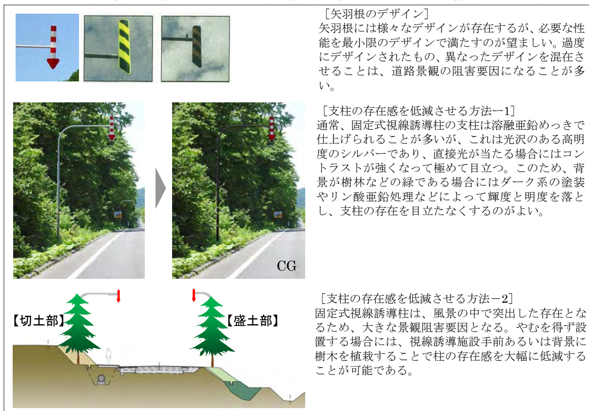
図 9.2 視線誘導柱の修景事例
