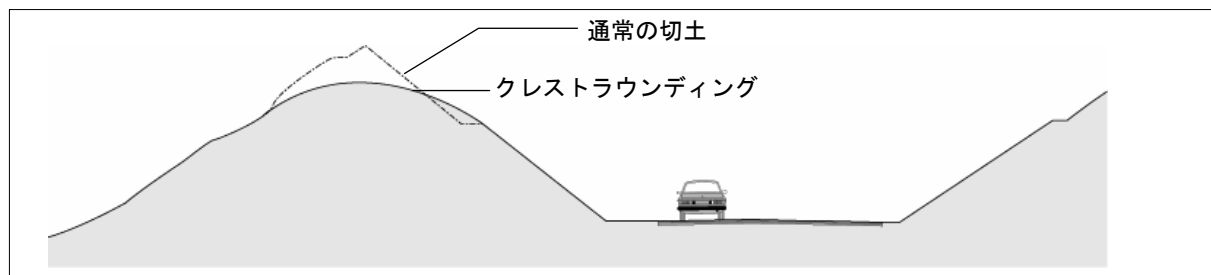
図 7.4 クレストラウンディングの事例
