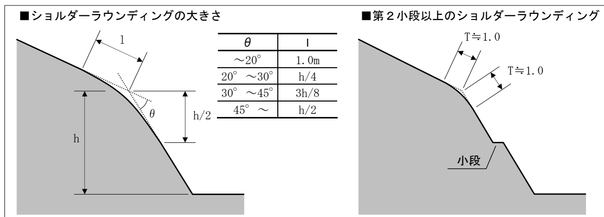
図 7.3 ショルダーラウンディング（出典：資料3）
