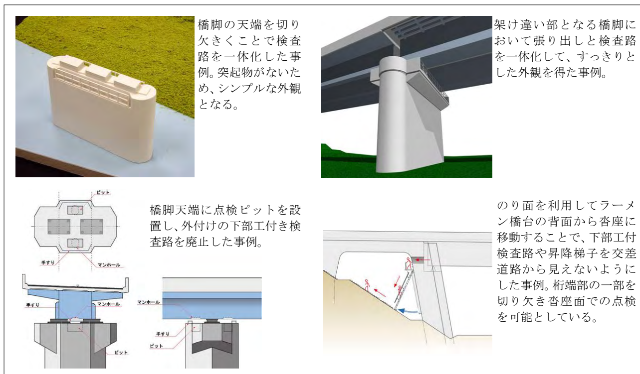
図 8.2.11 下部工付検査路を工夫した例
