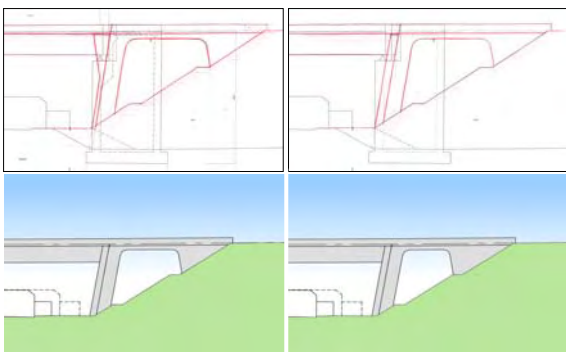
図 5.3.3 側面図による造形の検討（採用案は左下）
