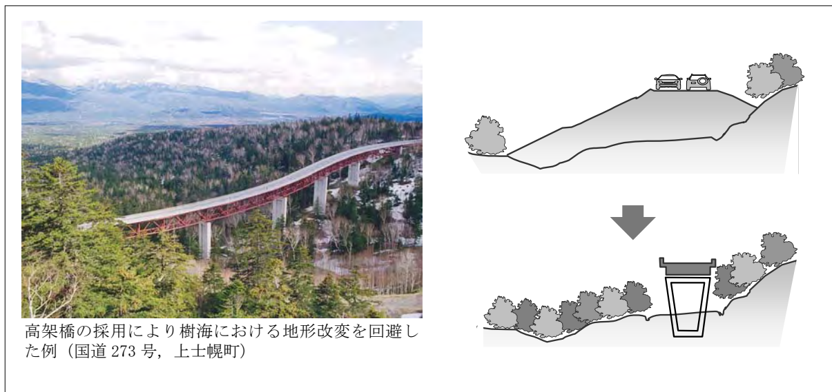
図 6.11 高架・橋梁による盛土のり面の回避
