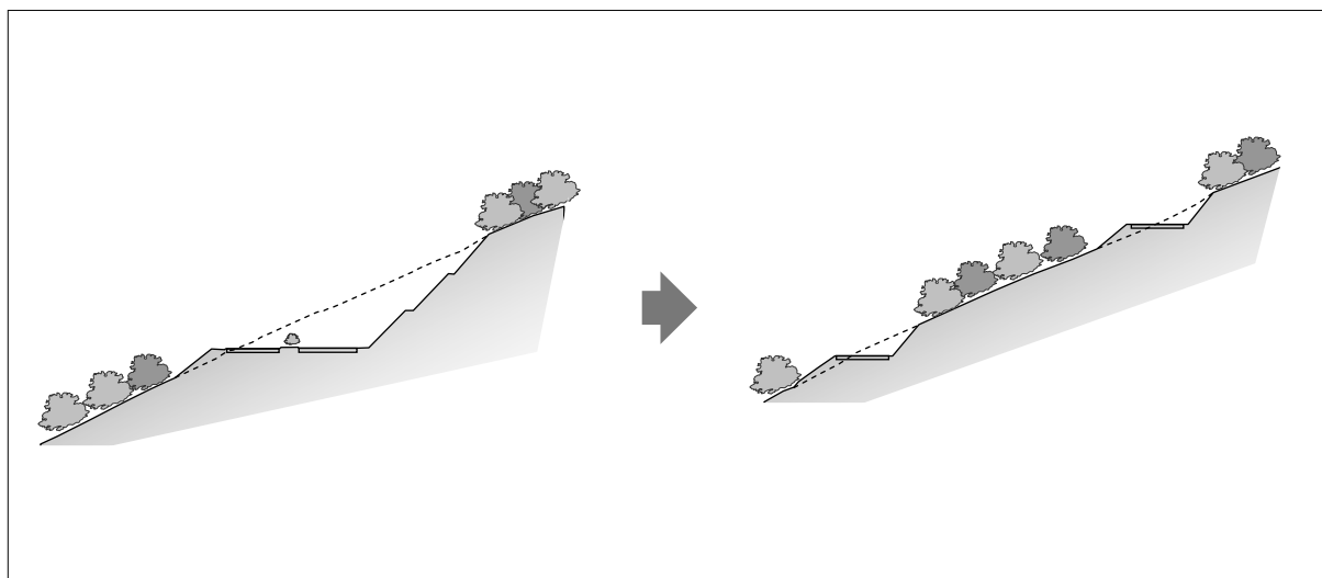
図 6.10 上下線分離方式
