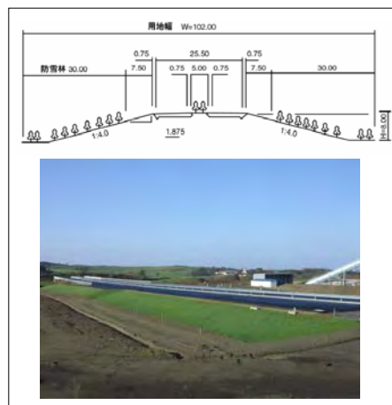
図 7.9 一般国道 40 号豊富バイパスにおける緩勾配盛土とその定規図
