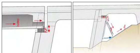
図 5.3.8 「見えない検査路」の概略図
