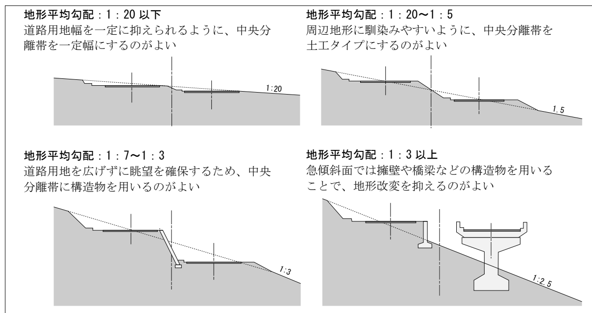
図 7.1 地形の勾配と上下線分離の構造（出典：資料 1 を一部修正）
