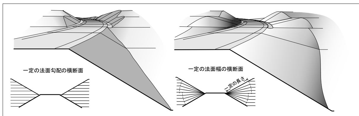
図 7.11 一定のり面勾配造成と一定のり面幅造成（出典：資料4）
