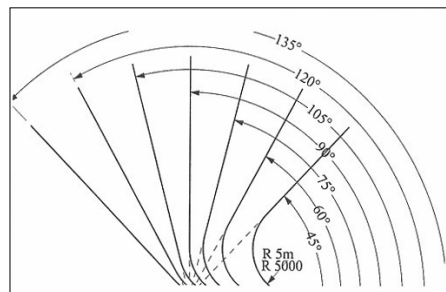
図 7.6 コンターラウンディング（出典：資料2）
