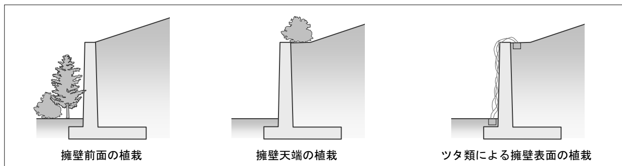
図 8.4.2 植栽による修景
