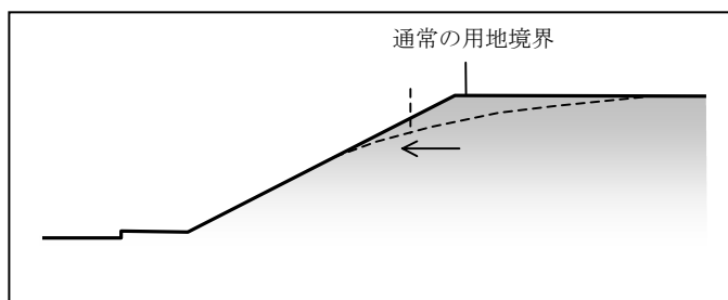
図 12.1.1 ゆるやかなラウンディングにより農地に返還される地形の造成
