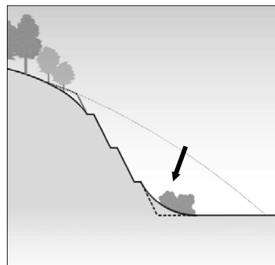
図 7.5 のり尻のラウンディング
