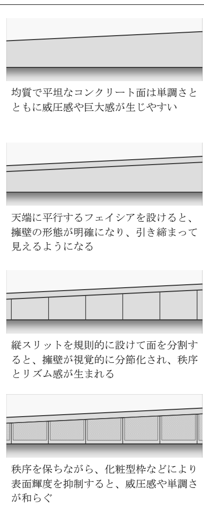
図 8.4.1 壁面のデザイン手法の例
