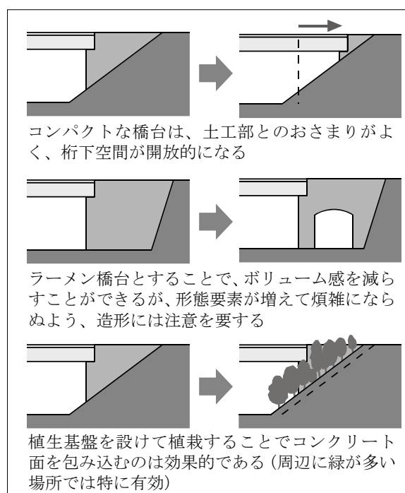
図 8.2.7 橋台検討時における配慮事項の例
