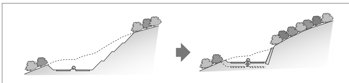
図 6.12 線形の微調整と擁壁の活用による切土のり面の縮小
