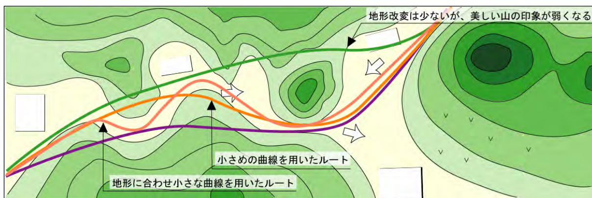
図 6.3 地形、地物と調和した線形計画（出典：資料 1）
