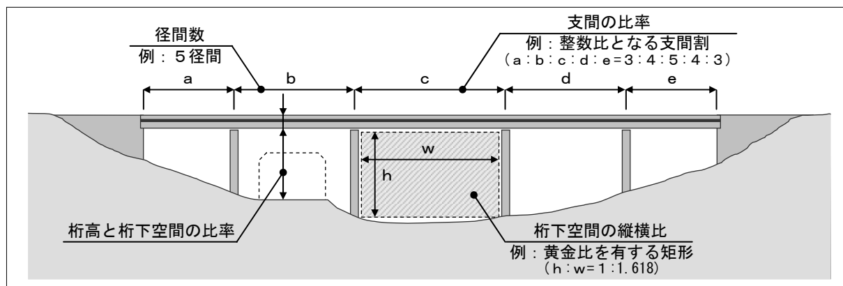
図 8.2.3 支間割の設定における着目点の例
