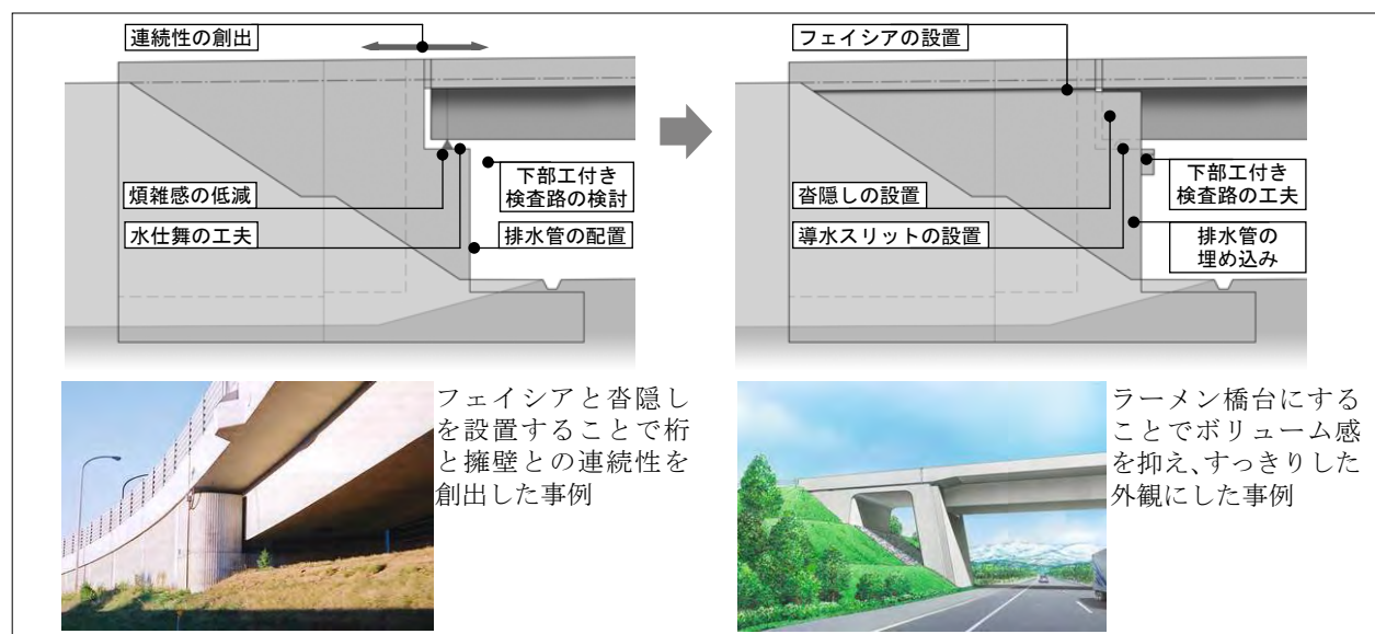
図 8.2.8 橋台における細部デザインの例
