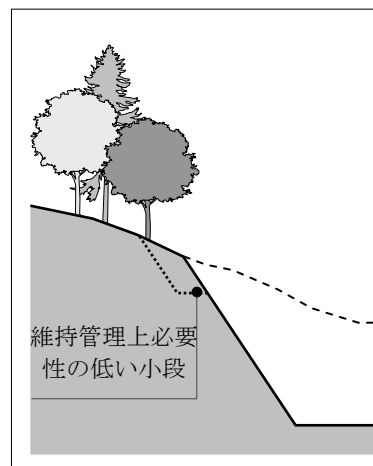
図 7.7 最上部の小段の削減
