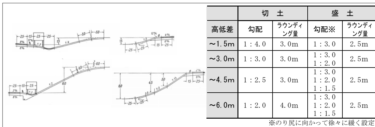
図 7.10 小規模切盛土における緩勾配化とラウンディング量の設定例（出典：資料 4）
