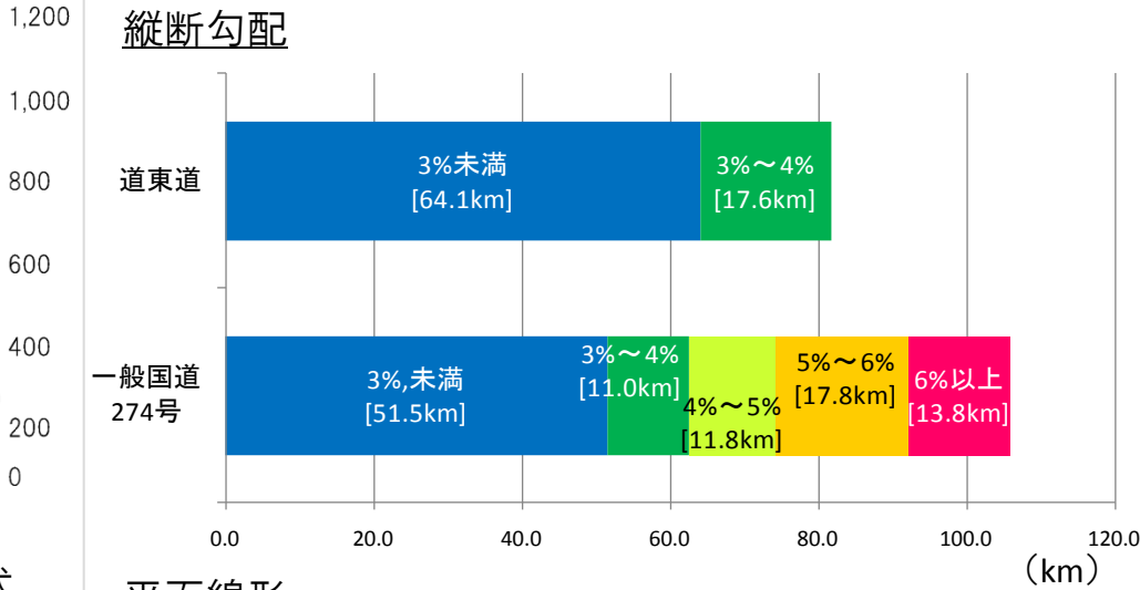
■道東道(夕張～十勝清水)と一般国道274号との線形比較
