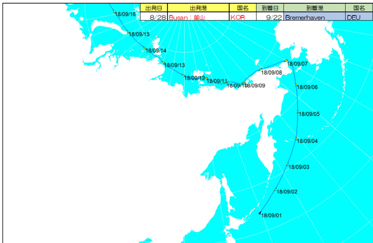
図-2 フルコンテナ船の航行事例
