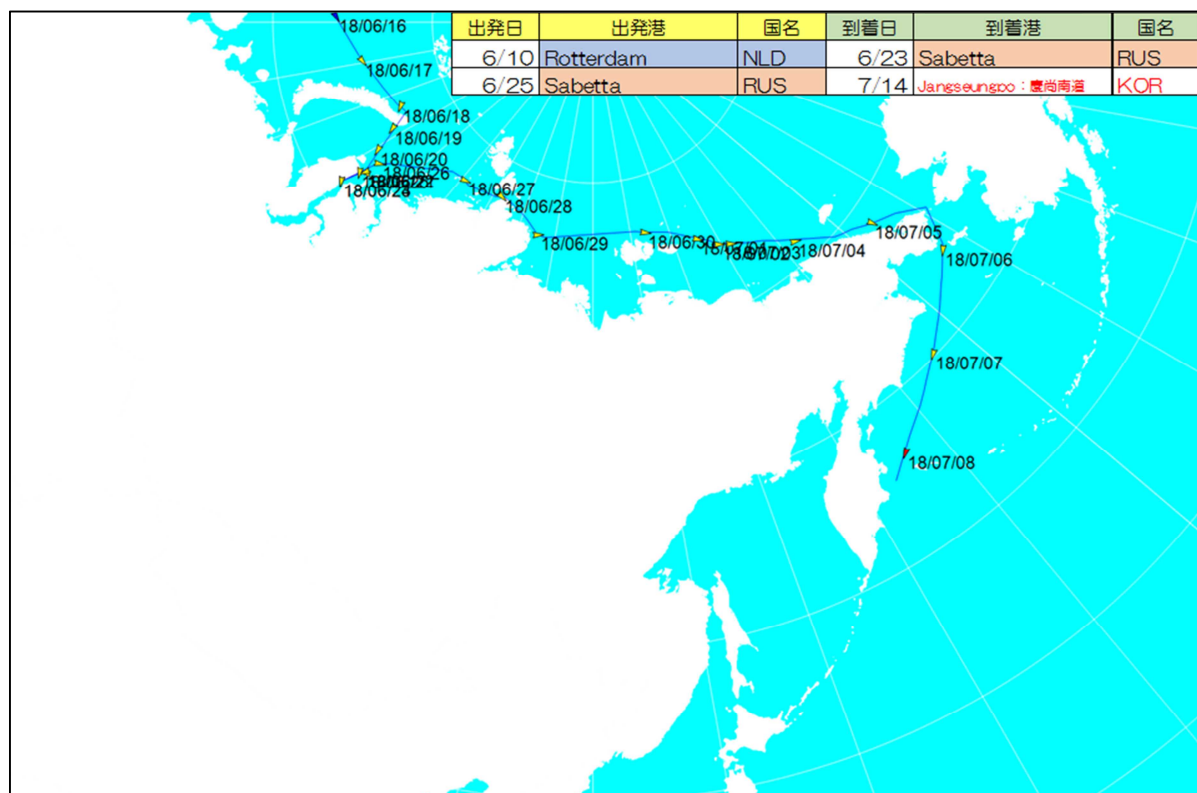
図-3 LNG タンカーの航行事例
