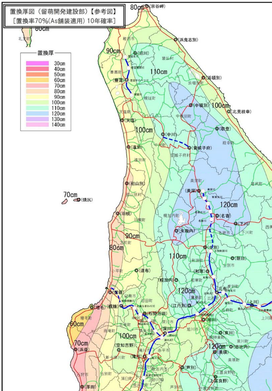
図4.1.17 置換率図（留萌開発建設部）【参考図】 [置換率70%(As舗装適用) 10年確率]
