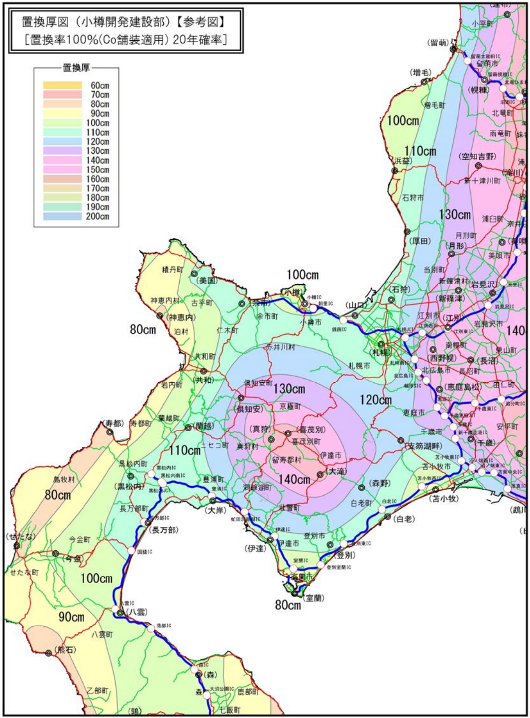
図4. 1. 23 置換率図（小樽開発建設部）【参考図】 [置換率100%(Co舗装適用) 20年確率]
