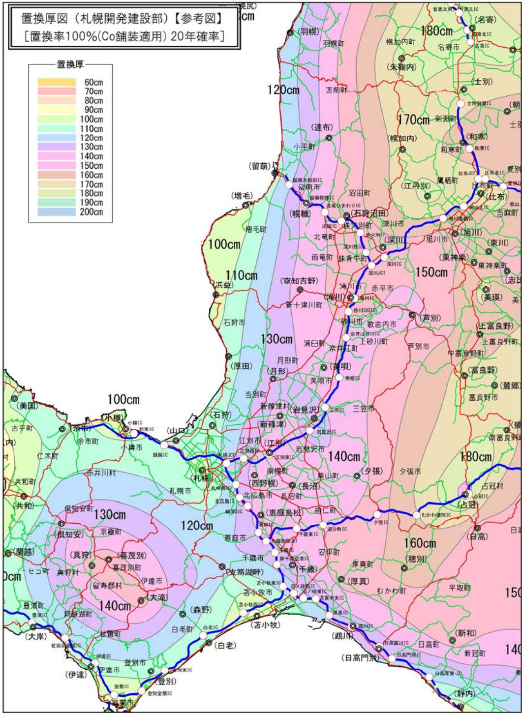
図4.1.21 置換率図 (札幌開発建設部) 【参考図】 [置換率100%(Co舗装適用) 20年確率]
