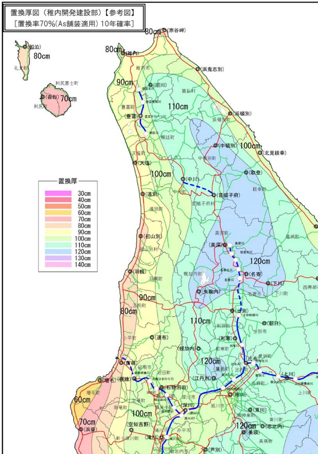
図4.1.19 置換率図（稚内開発建設部）【参考図】 [置換率70%(As舗装適用) 10年確率]
