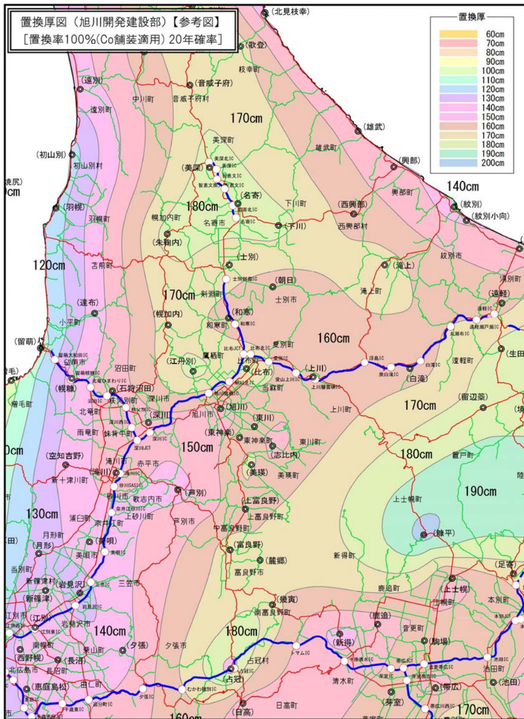
図4.1.24 置換率図 (旭川開発建設部) 【参考図】 [置換率100%(Co舗装適用) 20年確率]
