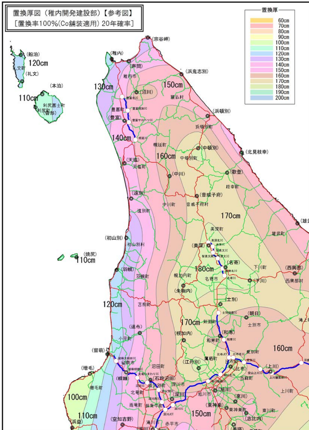
図4.1.30 置換率図（稚内開発建設部）【参考図】 [置換率100%(Co舗装適用) 20年確率]
