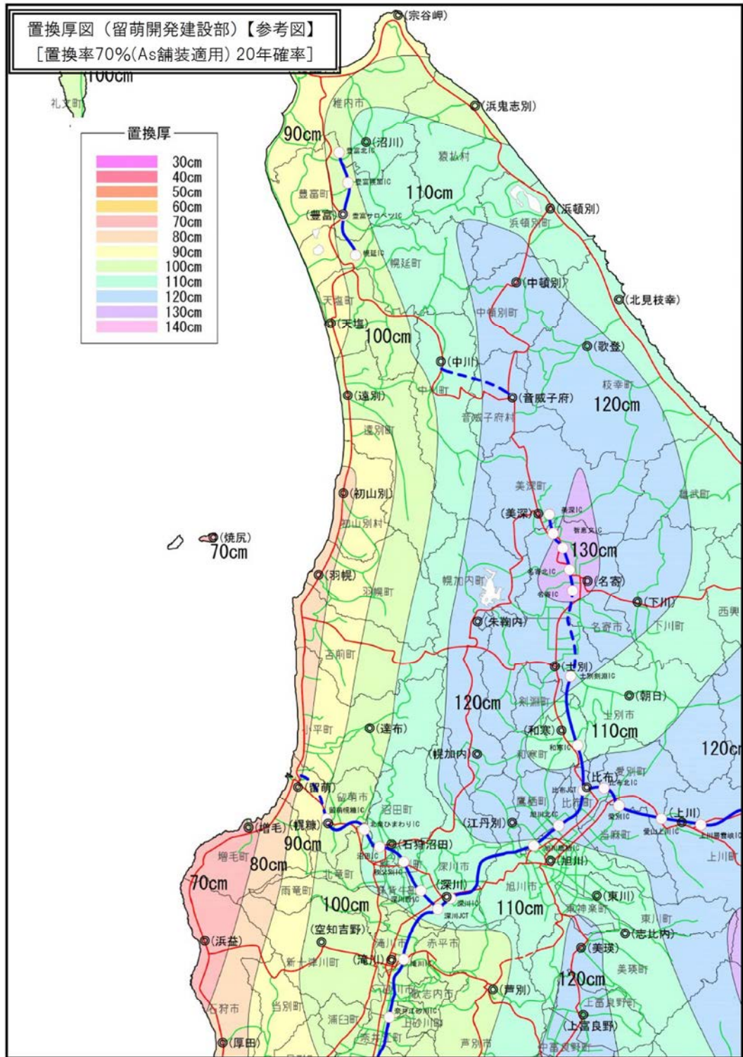
図4.1.18 置換率図（留萌開発建設部）【参考図】 [置換率70%(As舗装適用) 20年確率]
