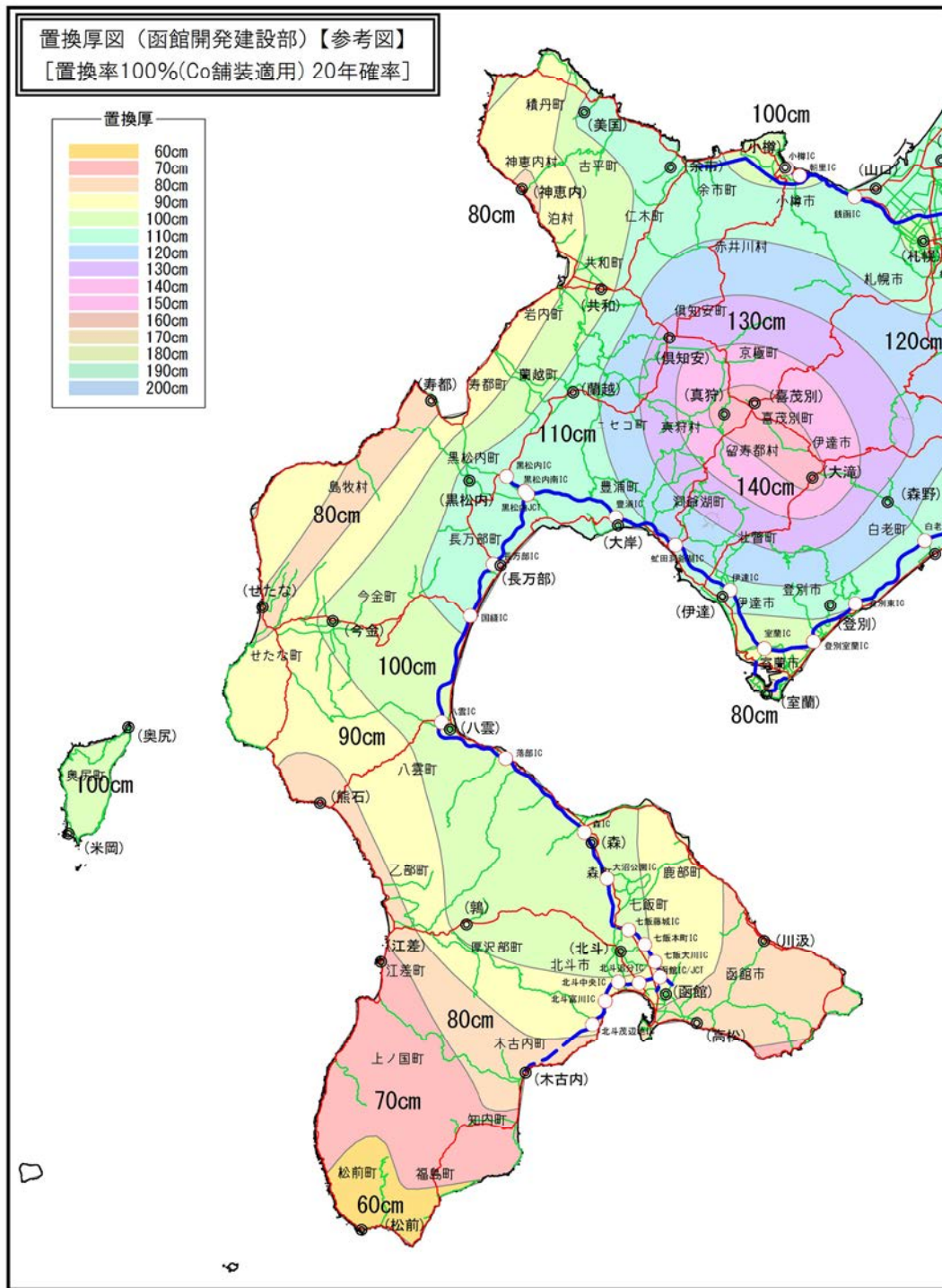
図4.1.22 置換率図(函館開発建設部)【参考図】 [置換率100%(Co舗装適用) 20年確率]
