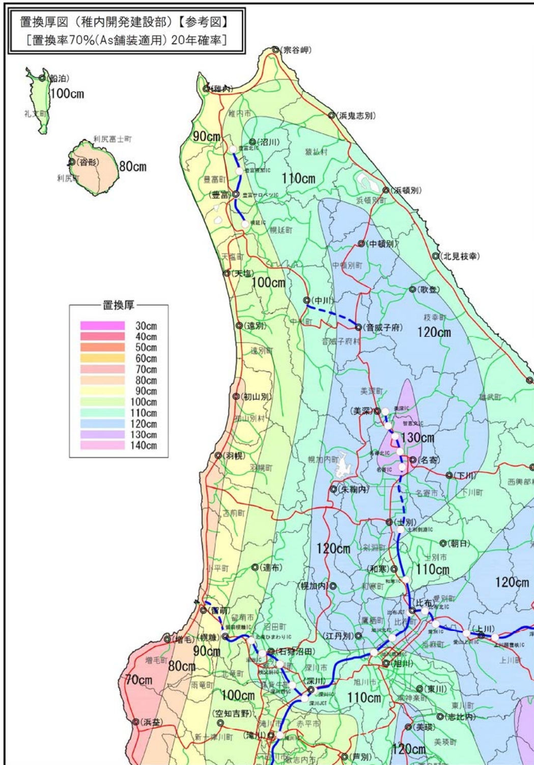
図4.1.20 置換率図（稚内開発建設部）【参考図】 [置換率70%(As舗装適用) 20年確率]
