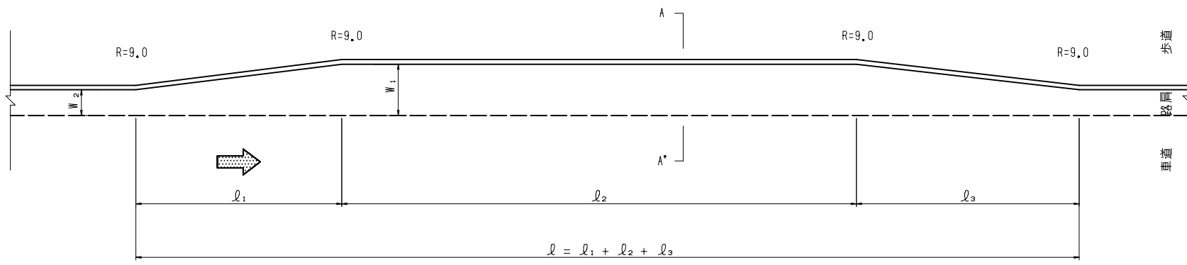
バス停車帯標準図
