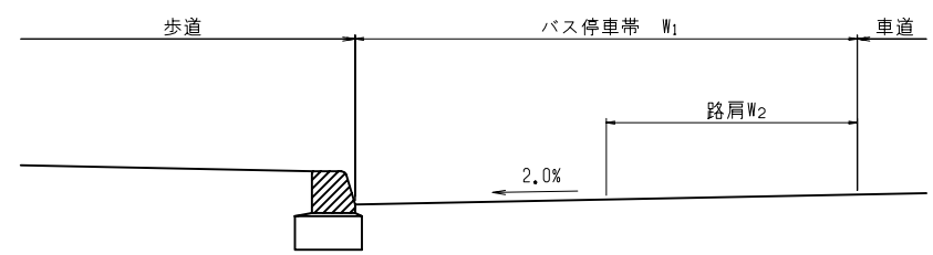
A - A' 断面図
