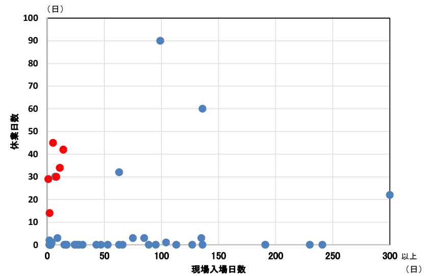
人身事故発生時の入場後経過日数と休業日数
