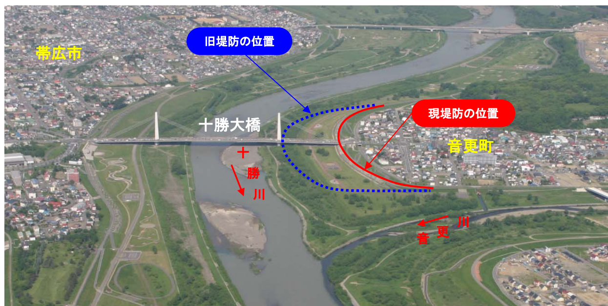
十勝川の引堤整備の事例
