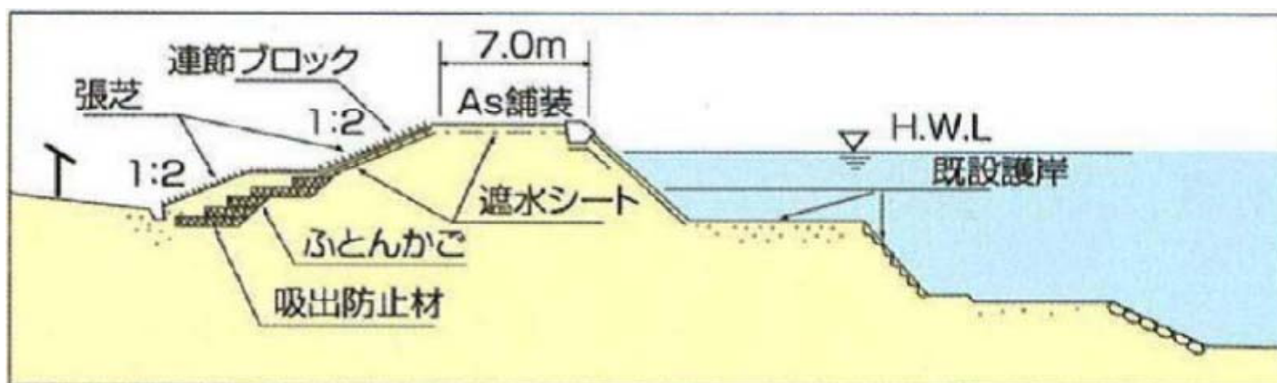
決壊しづらい堤防(アーマーレビー工法)
