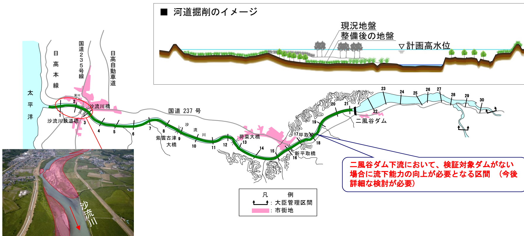
河川整備計画における河道掘削範囲の例
