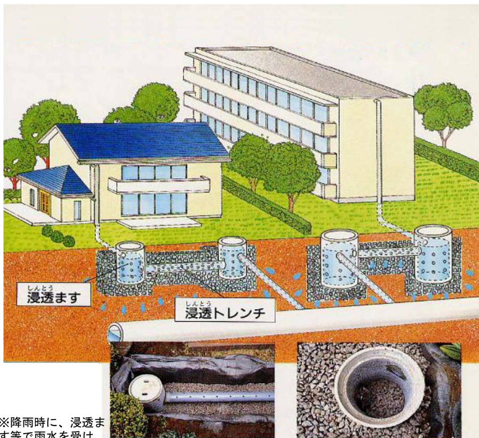
雨水浸透トレンチ
