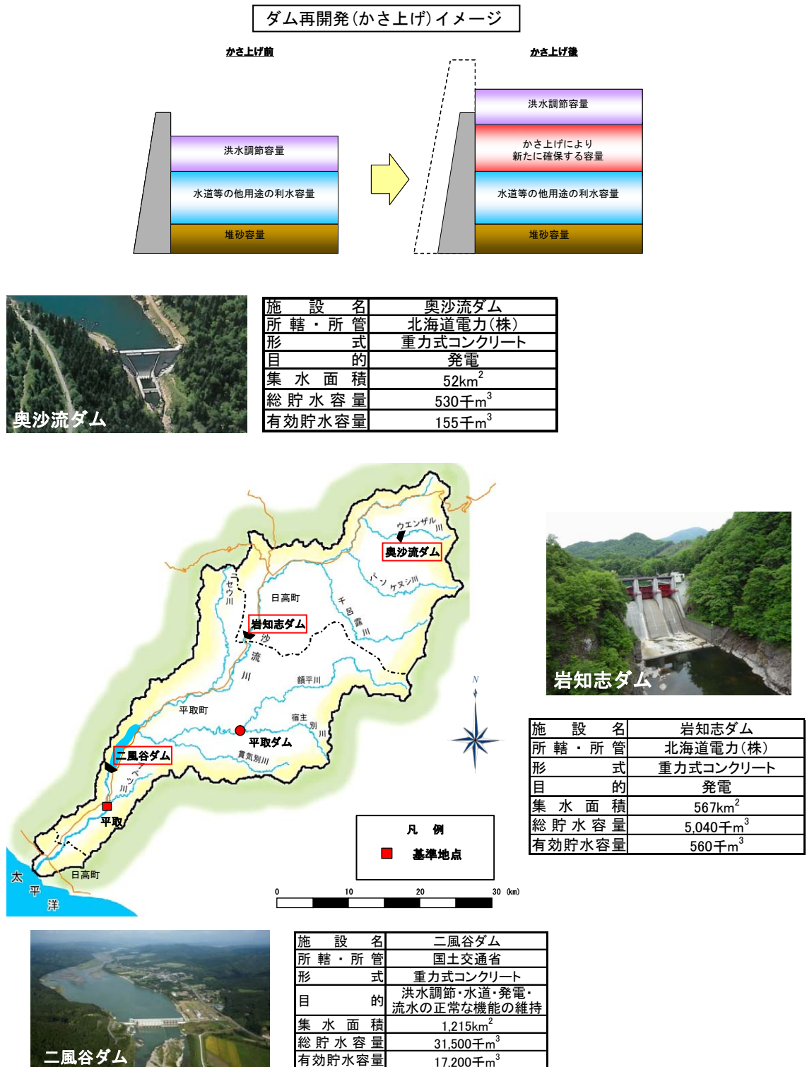
図 4.4-2 ダム再開発(かさ上げ・掘削のイメージ)
