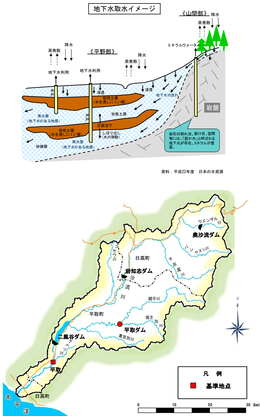
図 4.4-5 地下水取水のイメージ
