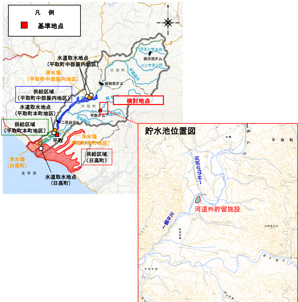
図 4.3-32 検討概要図
