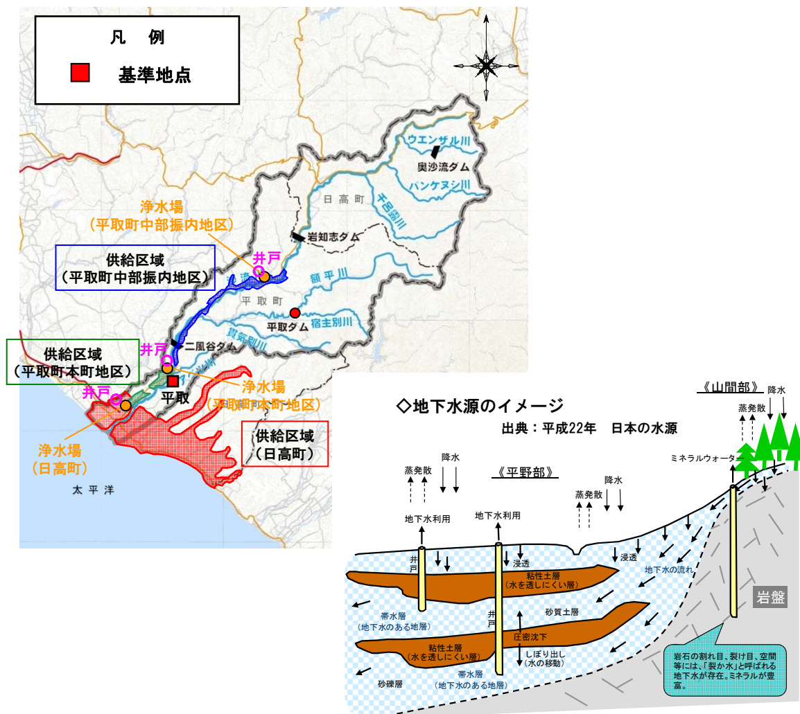
図 4.3-25 検討概要図
