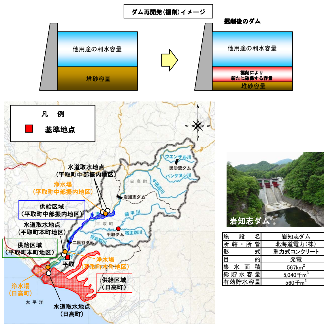
図 4.3-22 検討概要図
