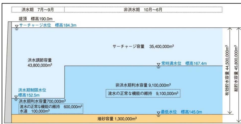
図 4.3-17 検討概要図
