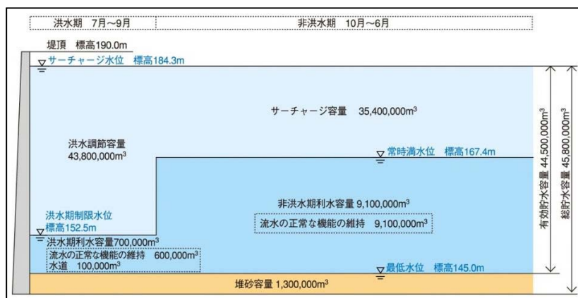
図 4.3-31 検討概要図
