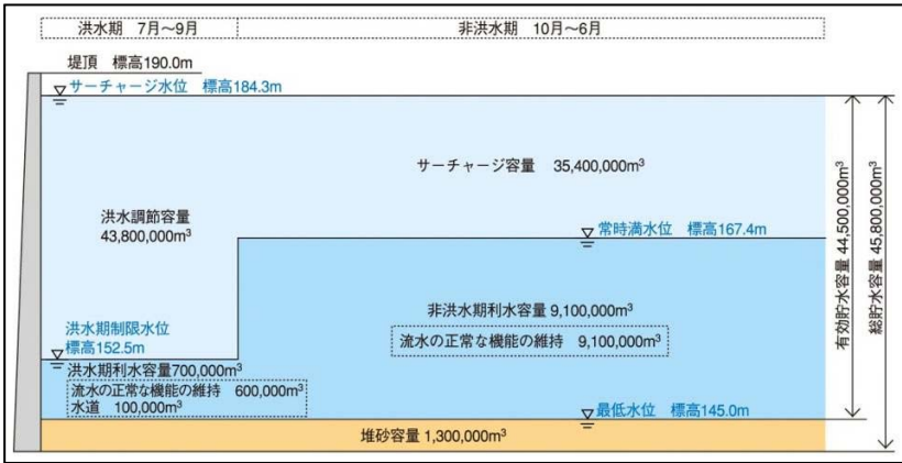
平取ダム貯水池容量配分図
