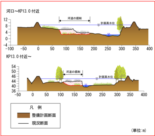
図 2-2 河道の掘削のイメージ図
