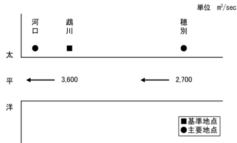
図 1-6 鵜川水系河川整備基本方針における計画高水流量配分図(単位: \text{m}^3/\text{s} )
