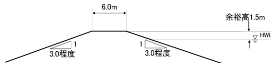
図 2-1 堤防整備の標準断面図(鵜川)
