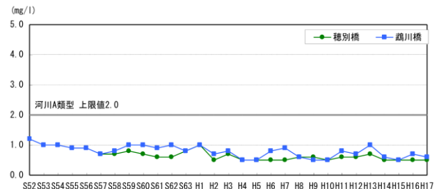
図 1-11 水質 (BOD75%値) の経年変化
