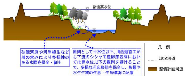
図 2-8 河道掘削のイメージ図
