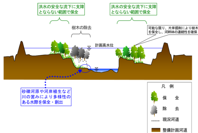
図 2-7 河畔林の保全、河岸の多様性の保全・創出イメージ図
