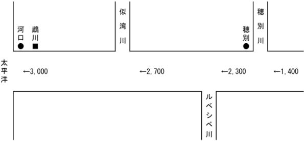
図 1-16 主要な地点における河道への配分流量(単位 : m³/s)
