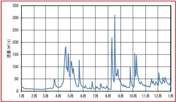
図 1-15 日平均流量の年変化(鵜川 基準地点鵜川、令和2年(2020年))
