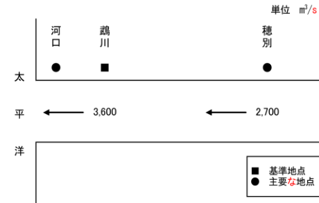
図 1-8 前河川整備基本方針(平成19年(2007年)11月)における鵜川計画高水流量配分図
