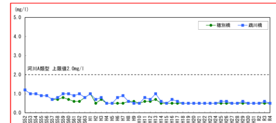
図 1-18 鵜川における水質 (BOD75%値) の経年変化
