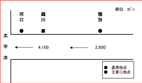
図 1-10 河川整備基本方針（令和6年（2024年）3月変更）における計画高水流量配分図
