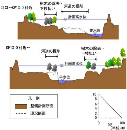
図 2-2 河道の掘削のイメージ図
