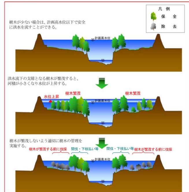
図 2-10 河道内樹木の管理イメージ図
