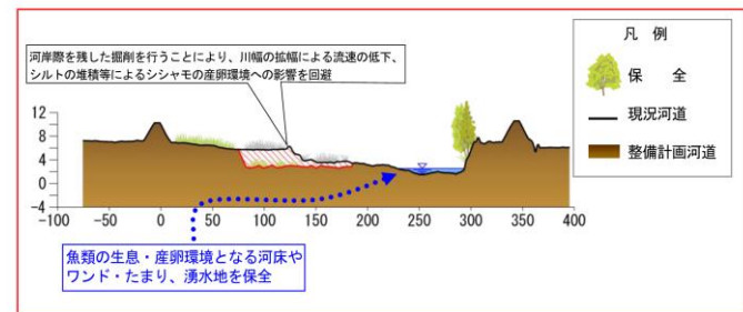
図 2-8 河道掘削のイメージ図
