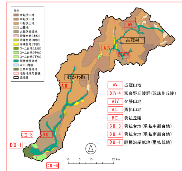
図 1-2 鵒川地形分類図
