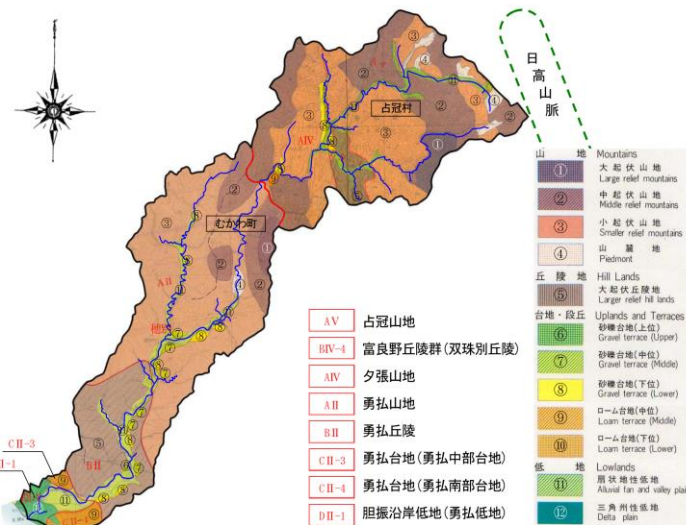
図 1-2 鵒川地形分類図
