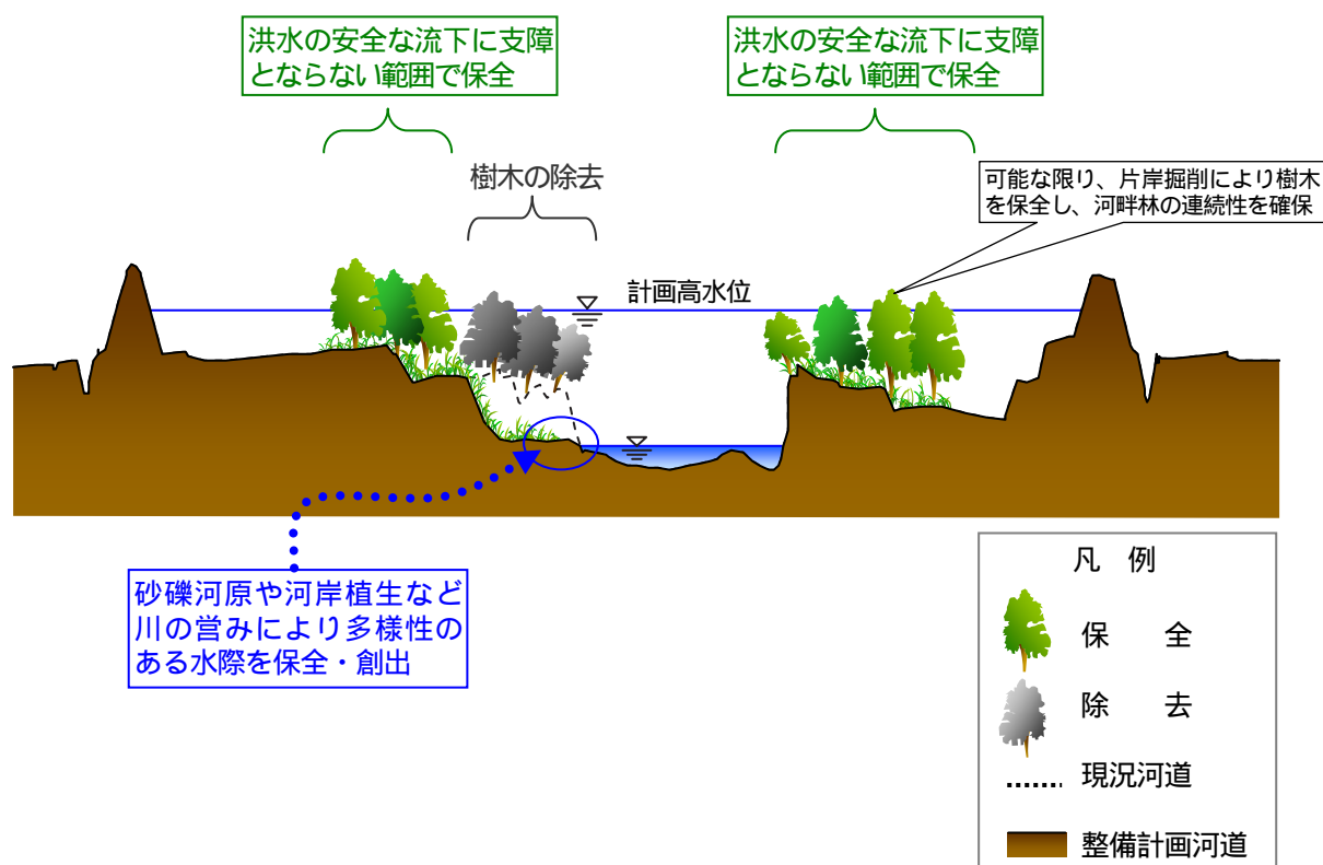
図 2-7 河畔林の保全、河岸の多様性の保全・創出イメージ図
