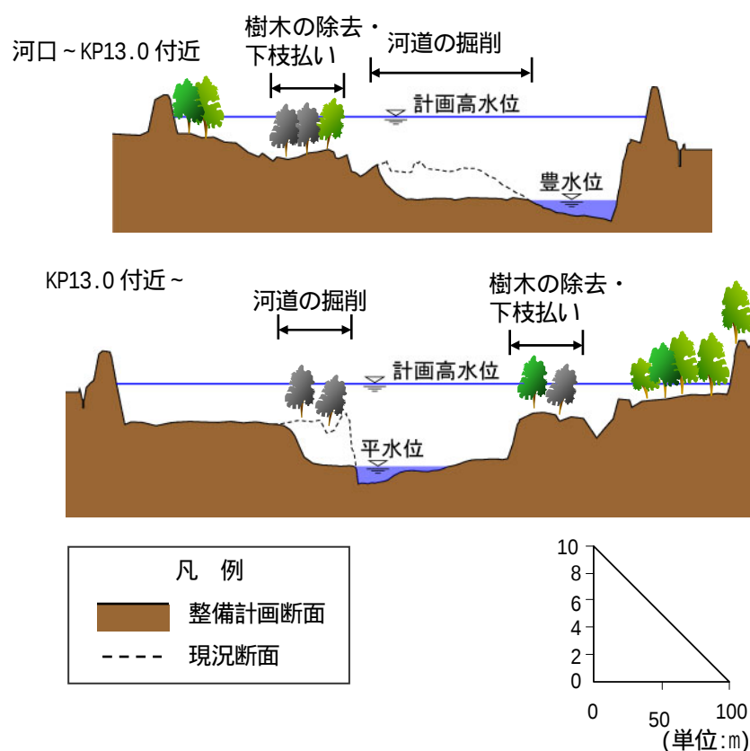
図 2-2 河道の掘削のイメージ図
