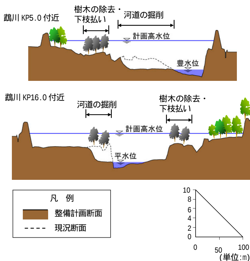
図 2-2 河道の掘削のイメージ図
