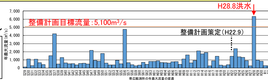
帯広観測所 年最大流量
