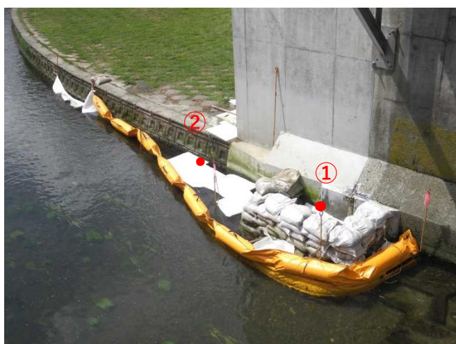
染み出し対策箇所①②の状況 (8/15撮影)
