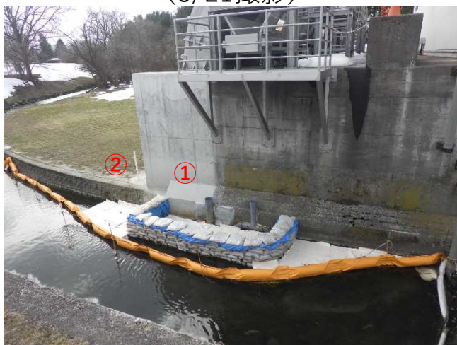
染み出し対策箇所①②の状況 (3/21撮影)
