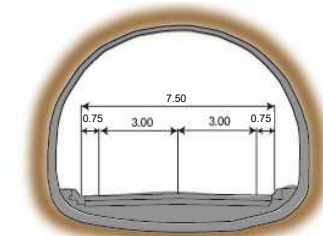
標準定規図
