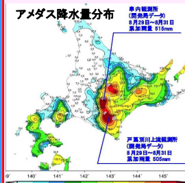
アメダス降水量分布 (平成28年8月29日1時～31日9時) 日本気象協会配付資料から転載
