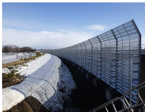
【防雪柵】
