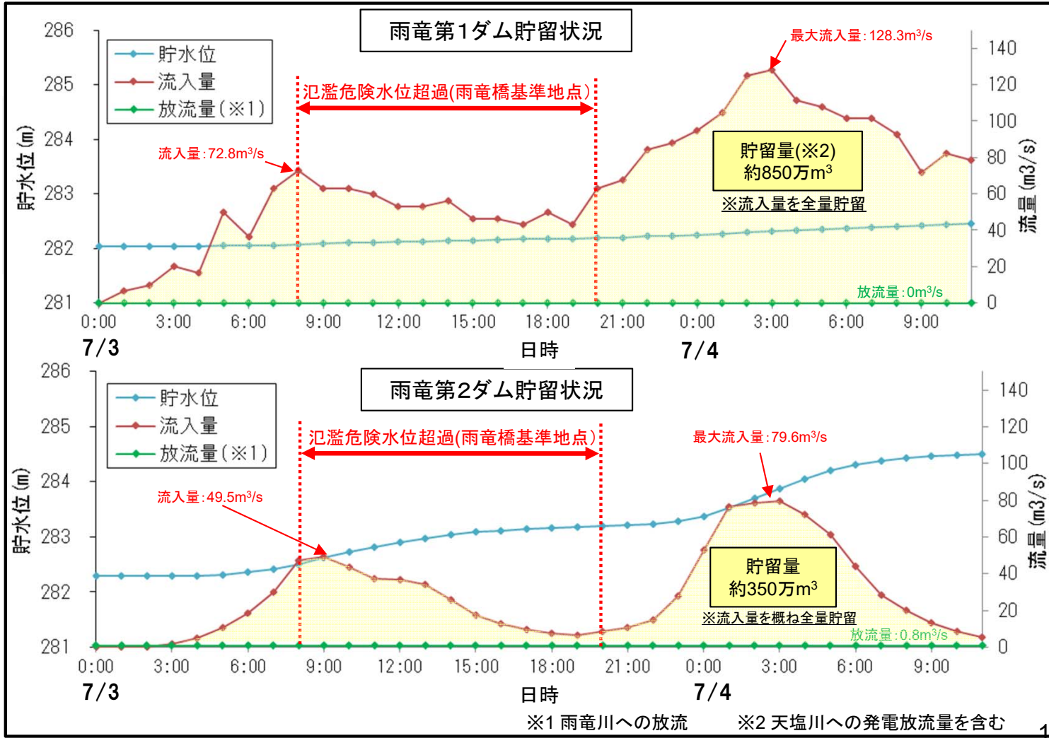
雨竜第2ダム (北海道電力株式会社)
