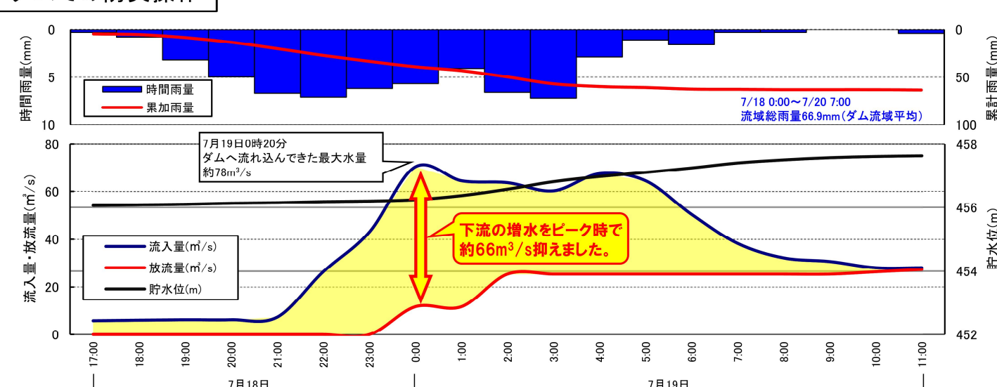
ダムでの防災操作
