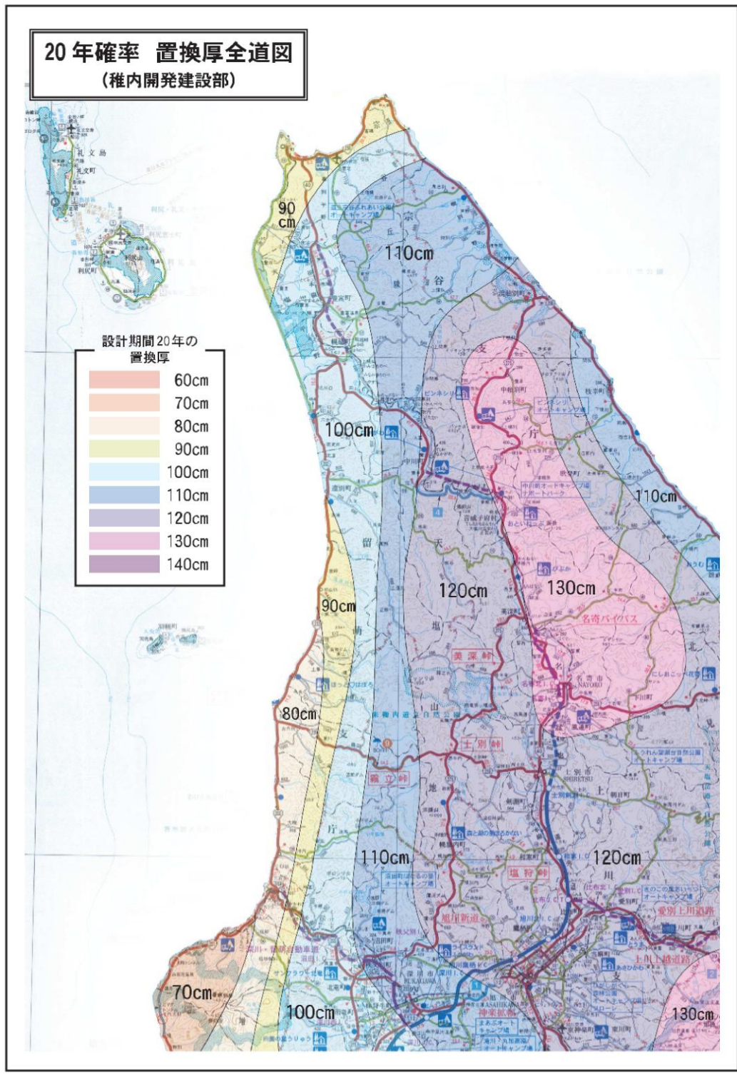
図4.1.10 20年確率置換厚全道図（稚内開発建設部）
