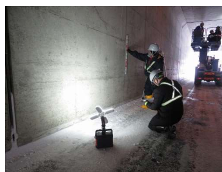
【大型カルバート点検】
