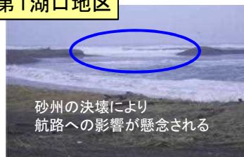
低気圧による砂州の決壊
