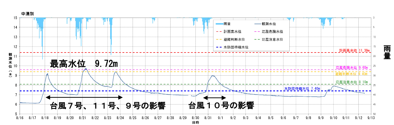
湧別川水系中湧別観測地点の水位状況
