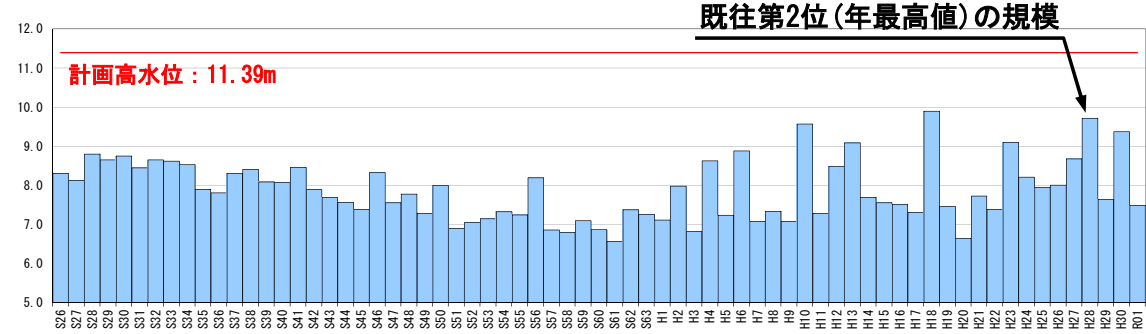
S26～R01年の年最高水位
