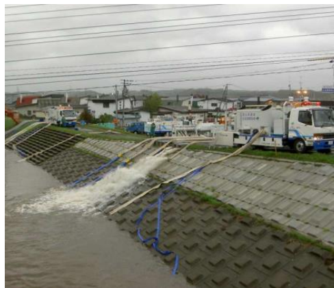
ポンプ車による内水排除の状況
