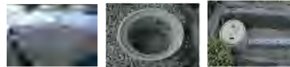
<雨水貯留浸透施設(左から貯留施設、浸透ます、浸透トレンチ)>
