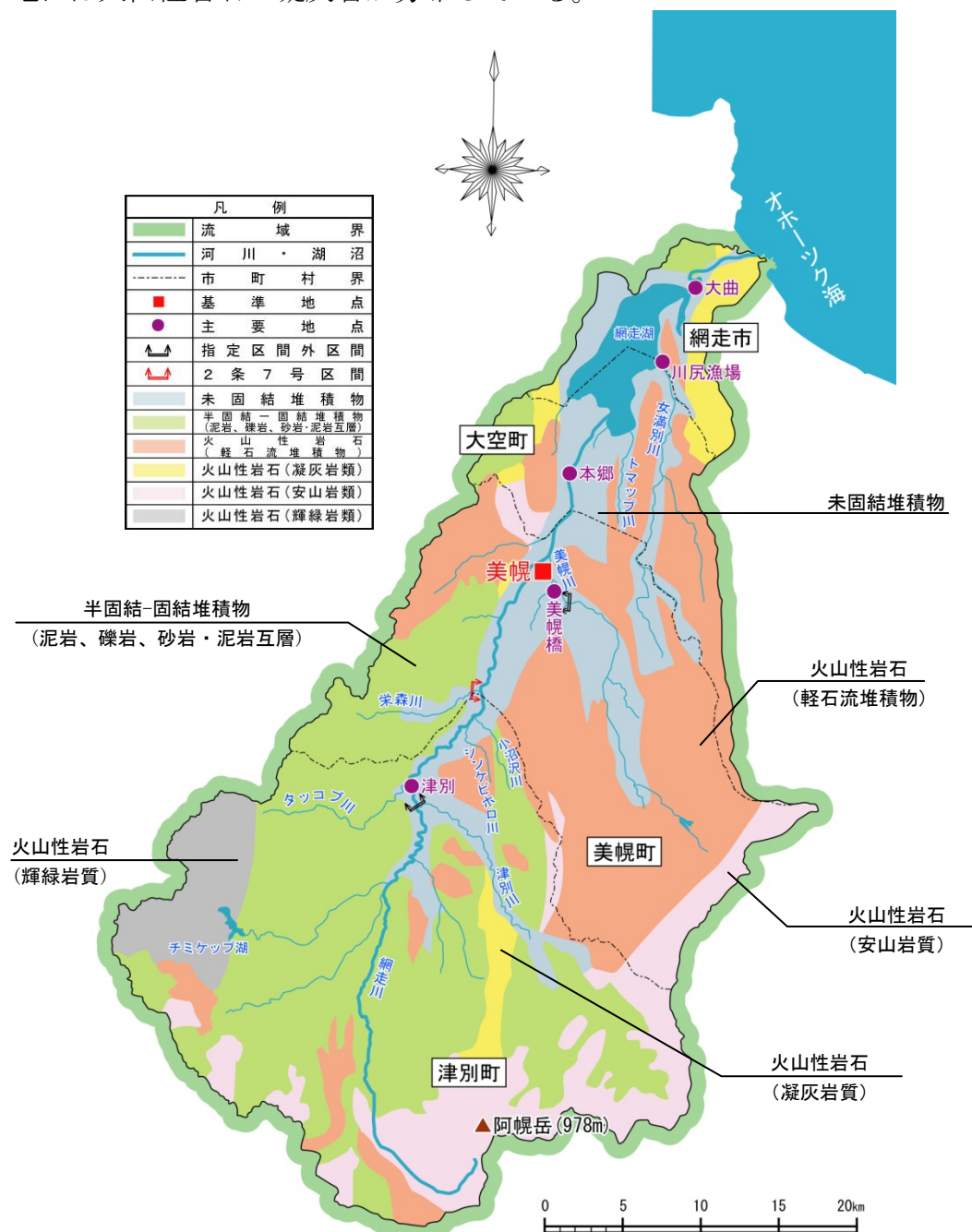
図 1-5 地質図
