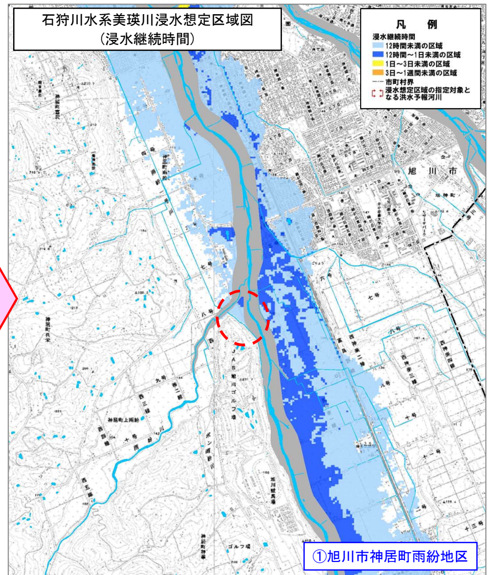
修正後(今回公表) 浸水想定区域図(浸水継続時間)
