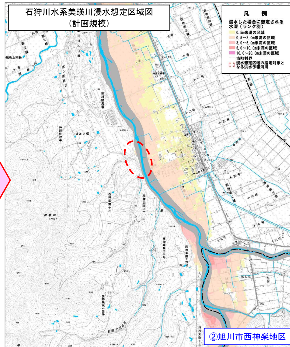
修正後(今回公表)浸水想定区域図(計画規模)
