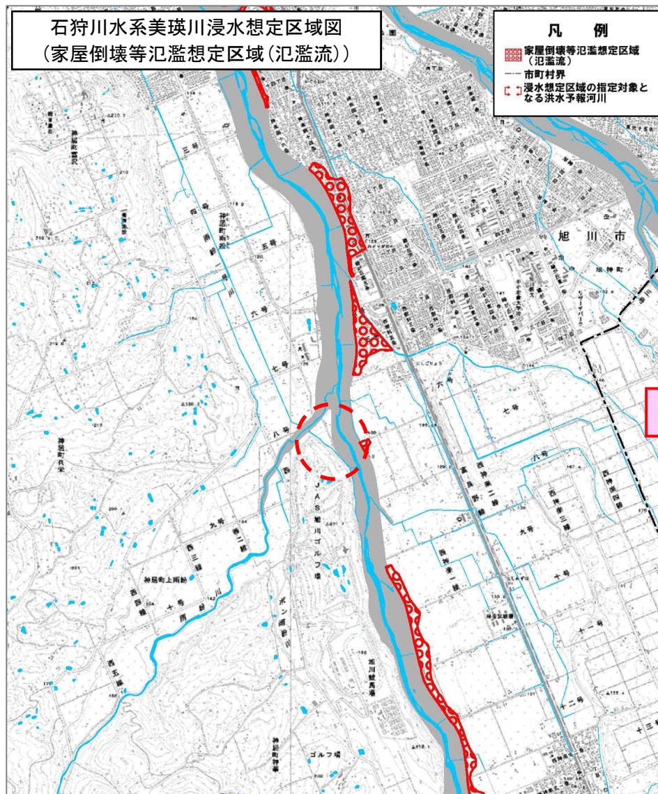
図-4 浸水想定区域図(家屋倒壊等氾濫想定区域(氾濫流))の比較図(美瑛川)
