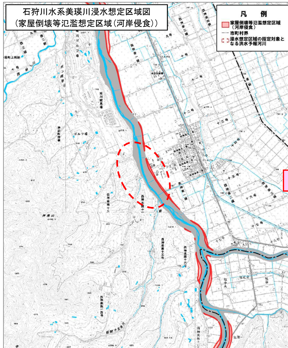
図-10 浸水想定区域図(家屋倒壊等氾濫想定区域(河岸侵食))修正前後の比較図(美瑛川)
