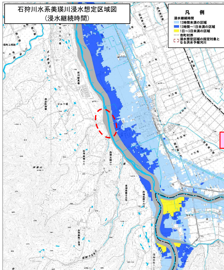
修正前(既公表) 浸水想定区域図(浸水継続時間)
