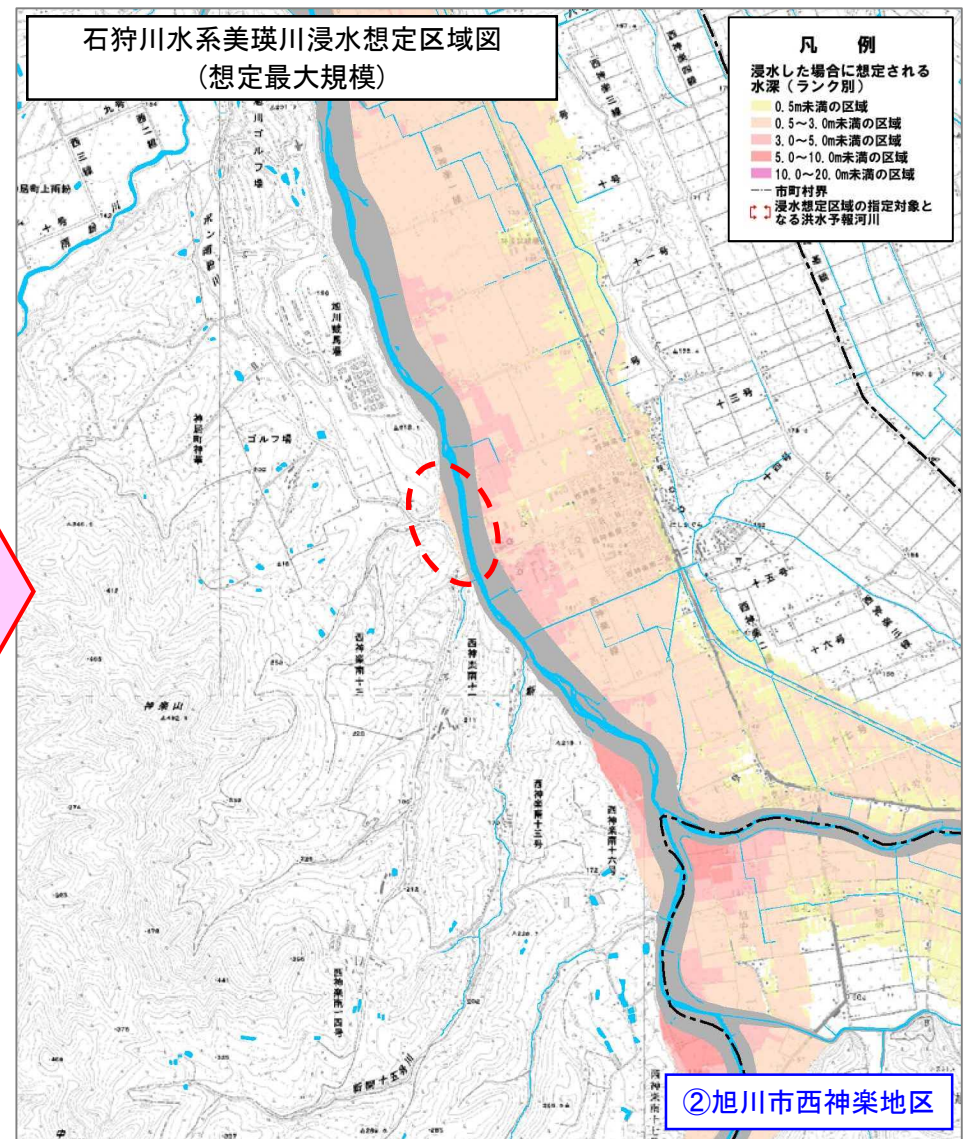
修正後(今回公表) 浸水想定区域図(想定最大規模)
