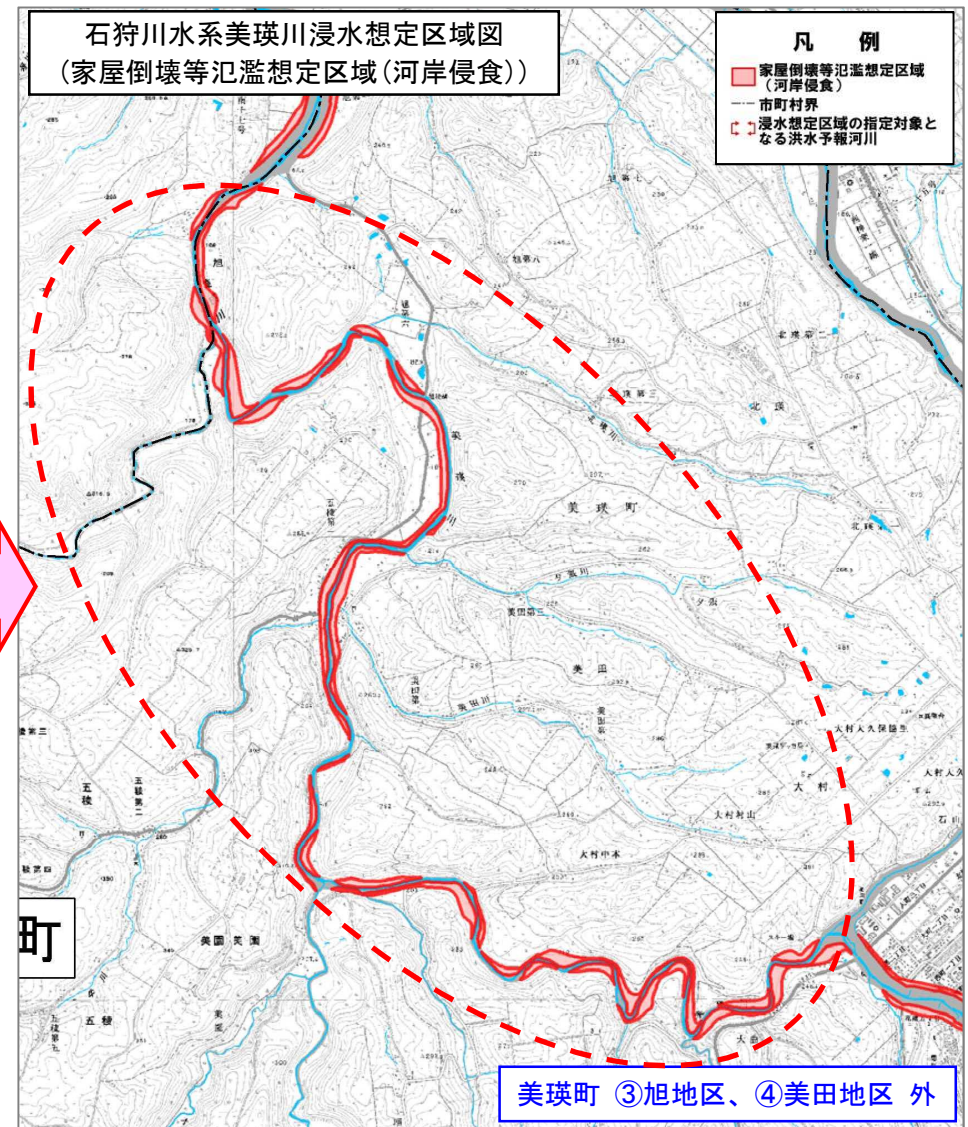
図-15 浸水想定区域図(家屋倒壊等氾濫想定区域(河岸侵食))修正前後の比較図(美瑛川)
