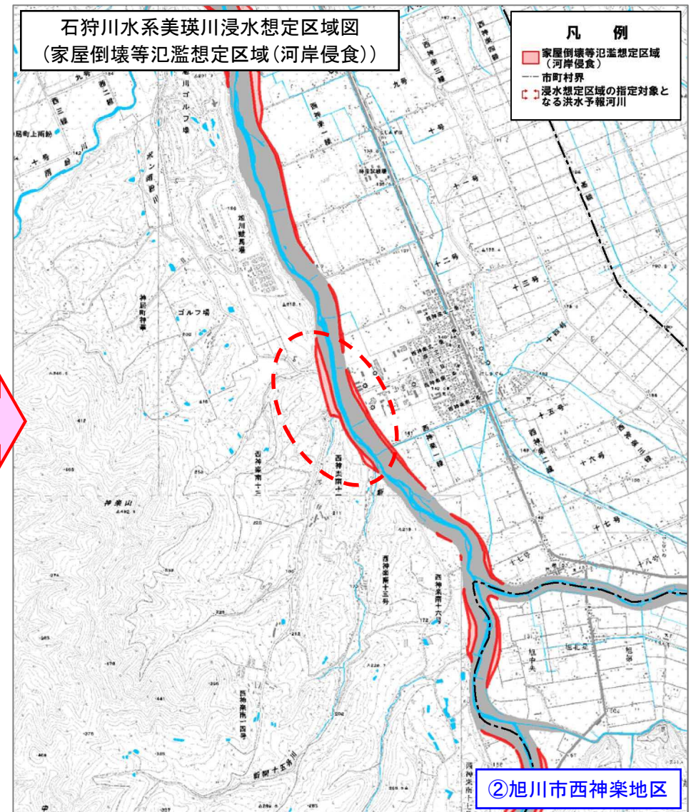
図-10 浸水想定区域図(家屋倒壊等氾濫想定区域(河岸侵食))修正前後の比較図(美瑛川)
