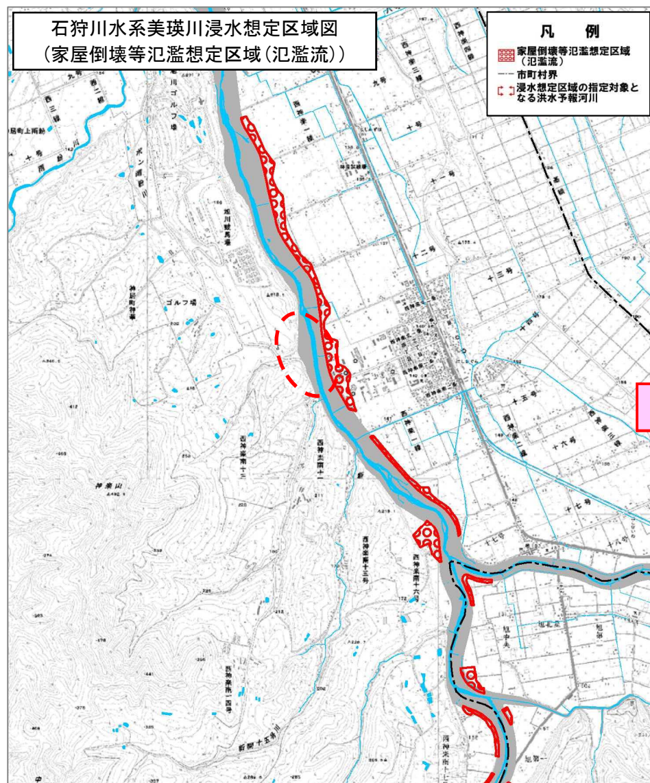
図-9 浸水想定区域図(家屋倒壊等氾濫想定区域(氾濫流))の比較図(美瑛川)
