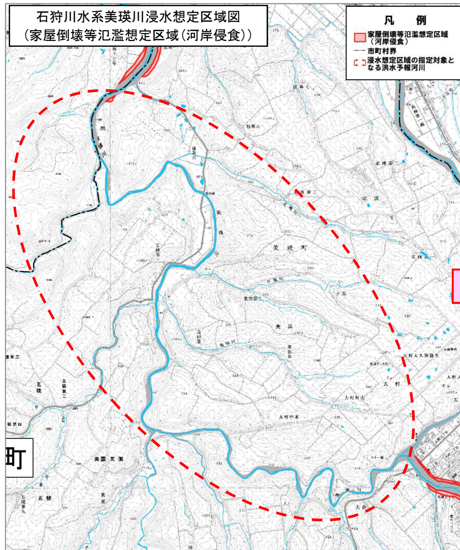
図-15 浸水想定区域図(家屋倒壊等氾濫想定区域(河岸侵食))修正前後の比較図(美瑛川)
