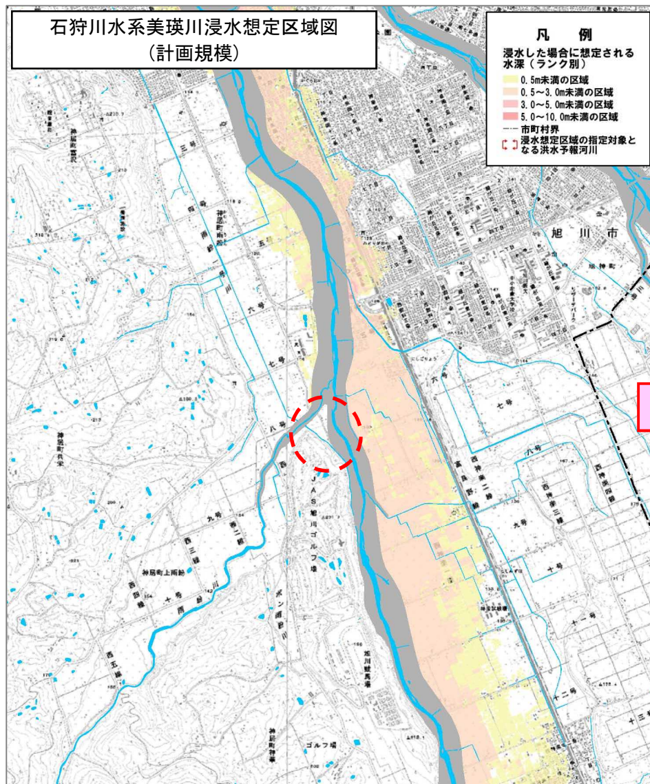
修正前(既公表)浸水想定区域図(計画規模)
