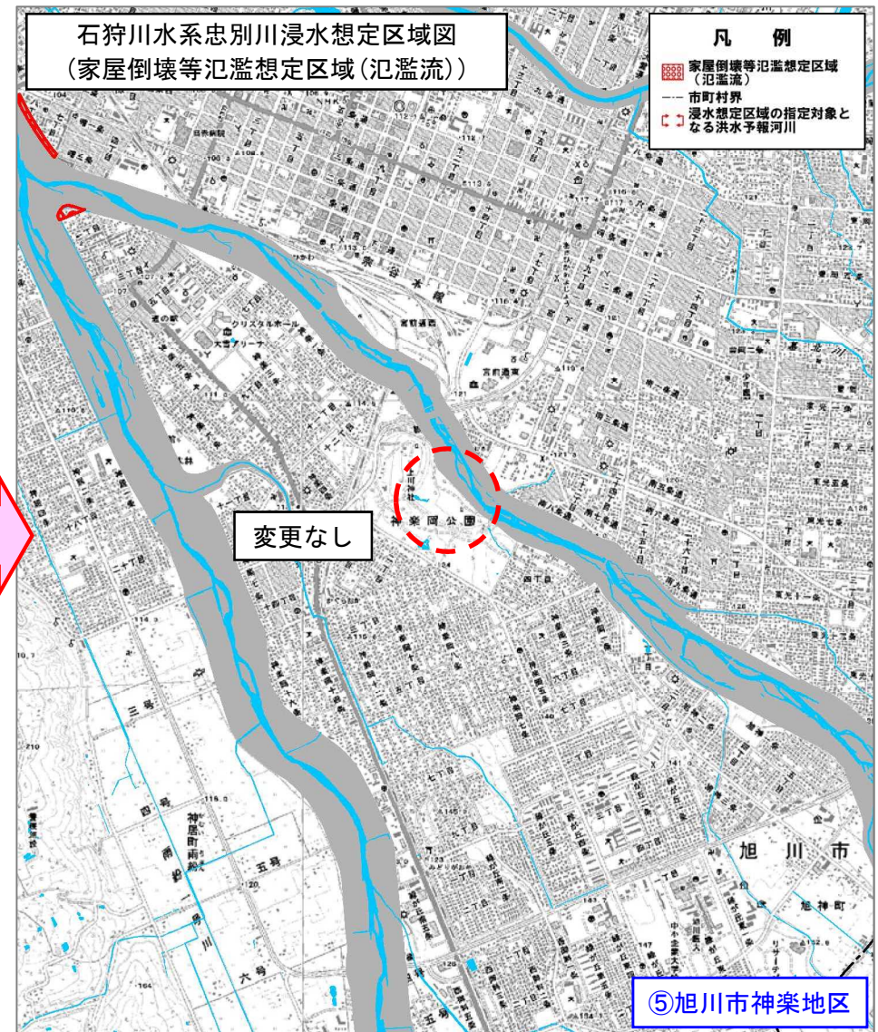
図-19 浸水想定区域図(家屋倒壊等氾濫想定区域(氾濫流))の比較図(忠別川)
