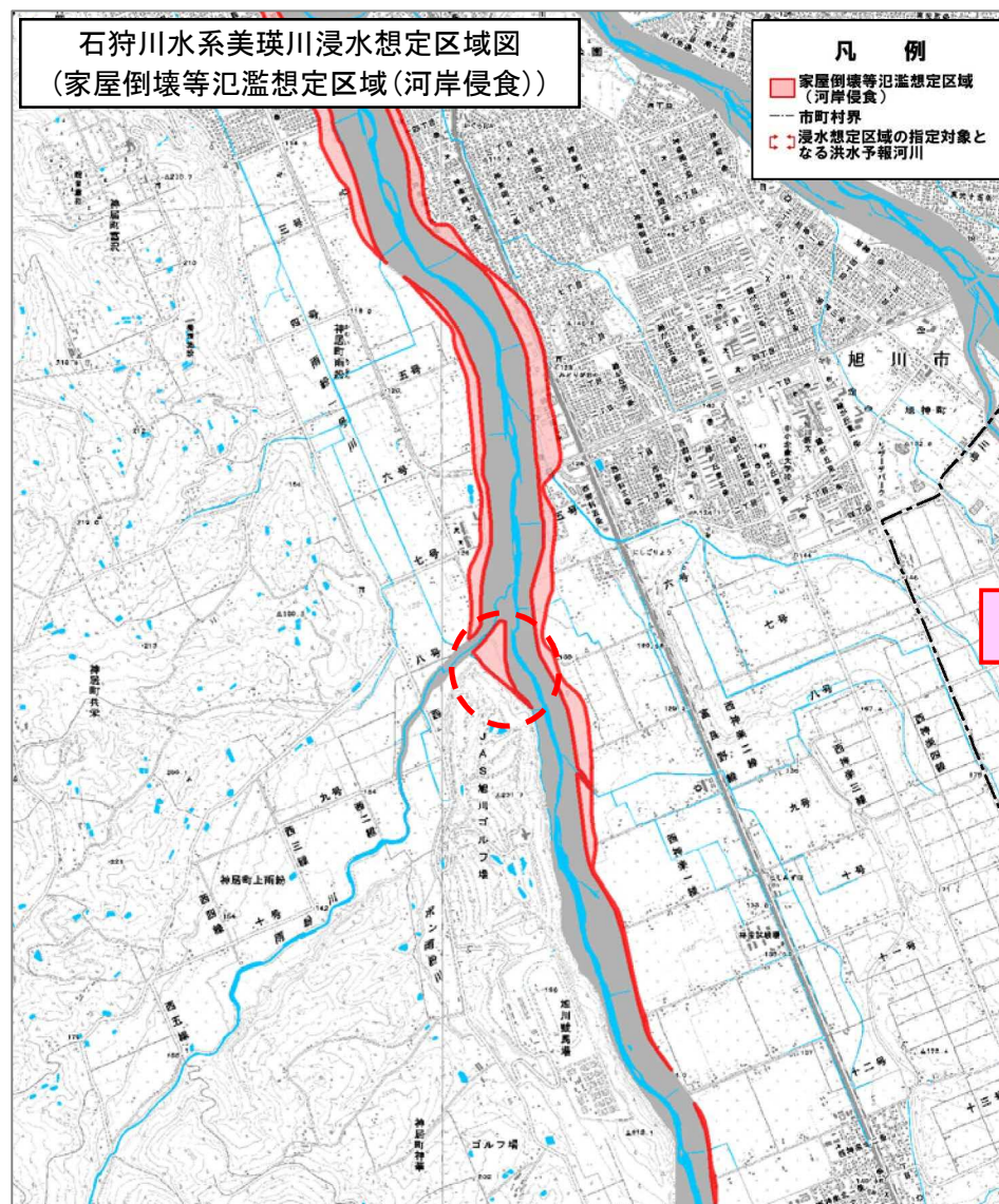
図-5 浸水想定区域図(家屋倒壊等氾濫想定区域(河岸侵食))修正前後の比較図(美瑛川)
