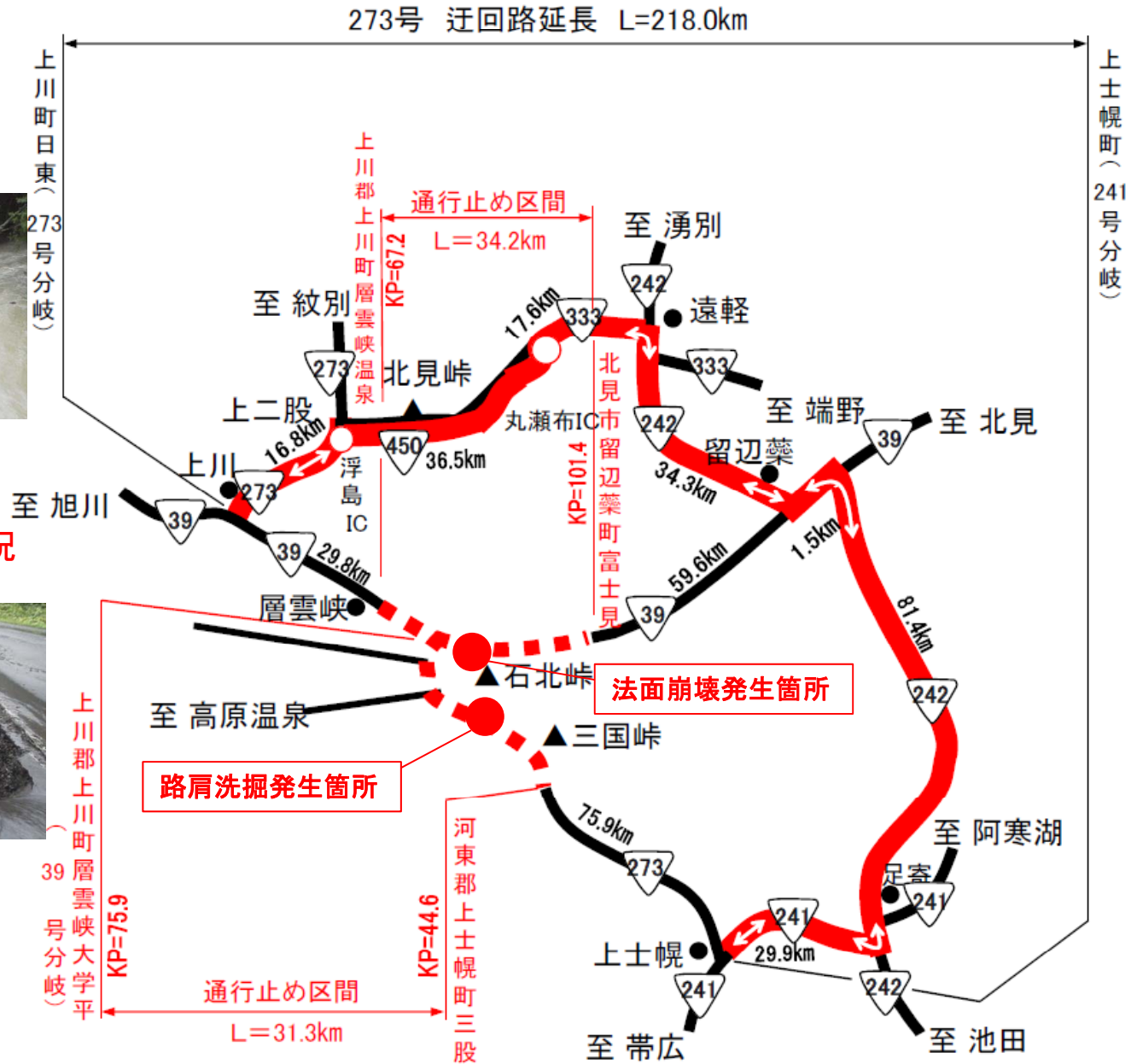
R39法面崩壊発生状況 (L=16m,H=3m,W=5m)
