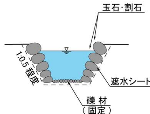
石積み水路
