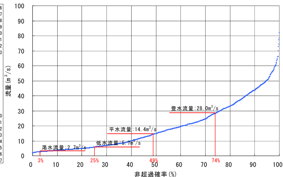
スモルト降下期中の発生流量確率
