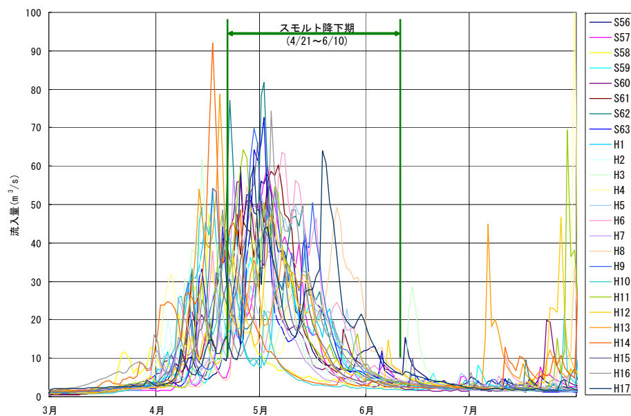
分水施設地点におけるスモルト降下期流量
