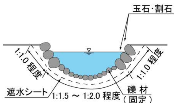
素掘り水路
