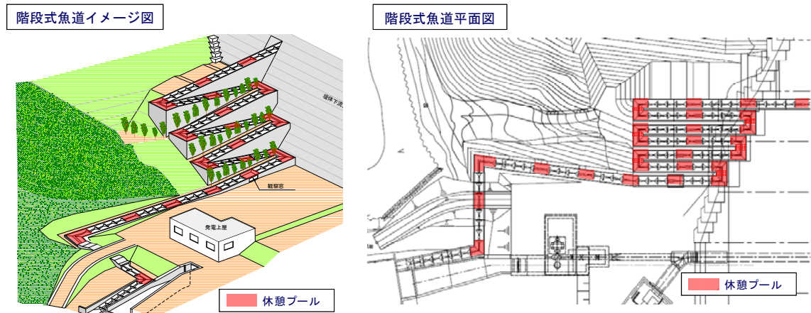
図- 20 階段式魚道のイメージ図と平面図
