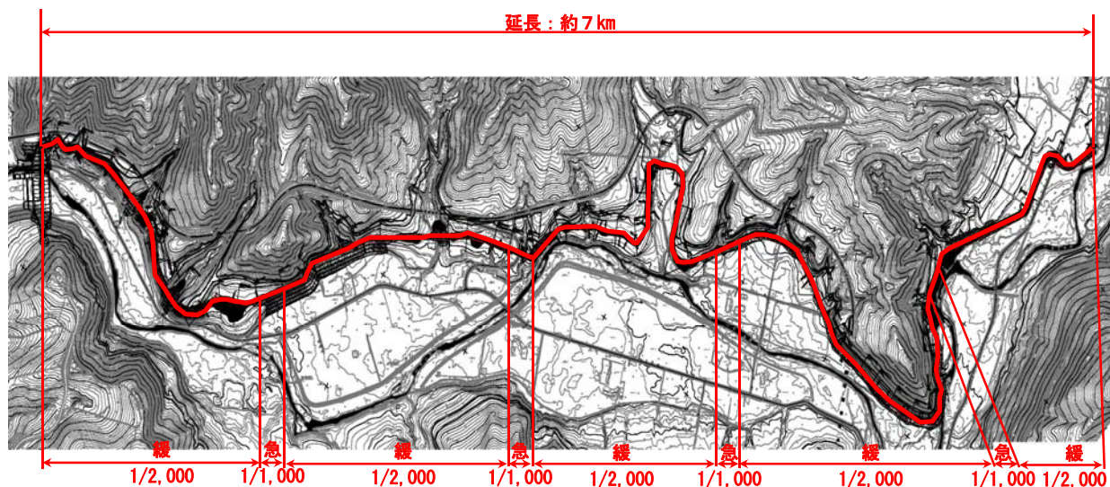
図- 22 パイパス水路の平面図と縦断勾配
