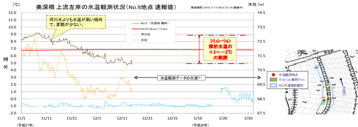
図- 63 水温観測地点（分流内礫州 No. 9）とシミュレーション解析結果との水温比較
