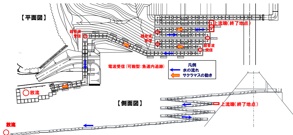
図- 52 階段式魚道 サクラマス遡上調査 位置図 (イメージ)
