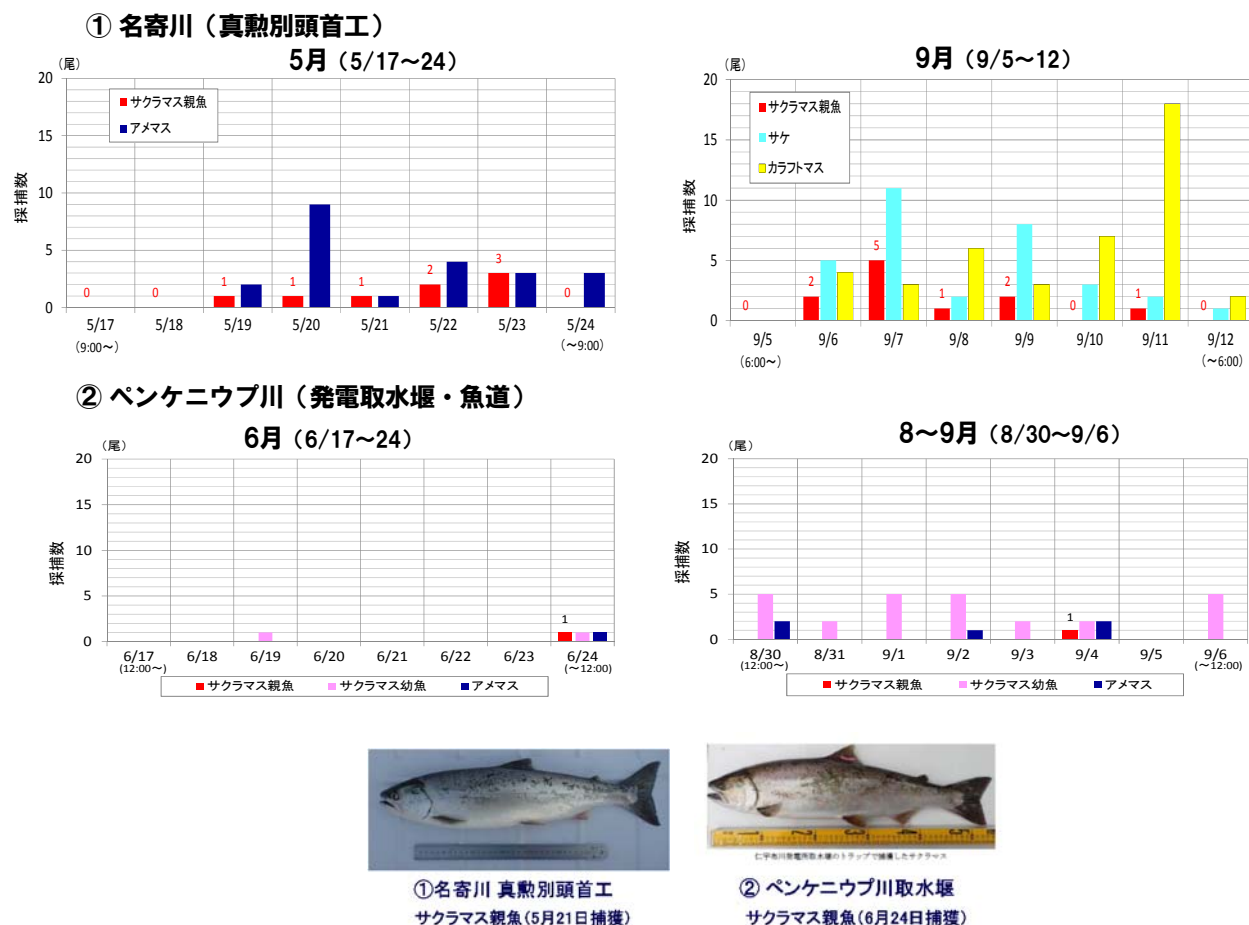
図-8 名寄川の頭首工及びペンケニウプ川取水堰における魚道トラップ調査結果
